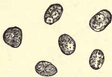
Fig. 37.— Sacch. ellipsoïdeus : development of spores ( \times 400 diam.).
