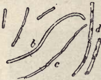
Fig. 83.—Malaria bacillus (Klebs and Cecci).
