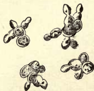
Fig. 38.— Sacch. ellipsoïdeus : germination of spores ( \times 400 diam.).
