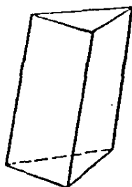
斜角柱
