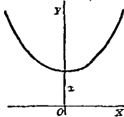
懸鏈線 CATENARY
