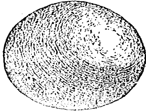
橢圓體
