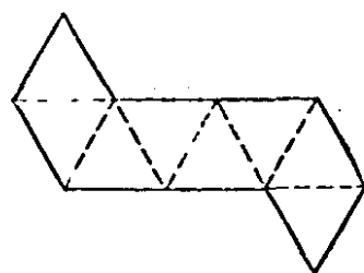
正八面體
