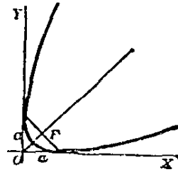
拋物線 PARABOLA
