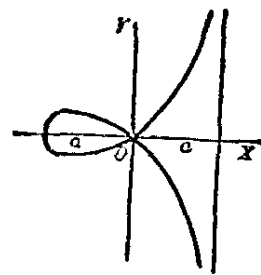
環索線 STROPHOID
