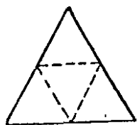
正四面體
