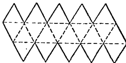
正二十面體
