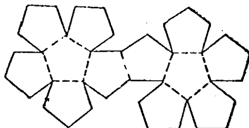
正十二面體
