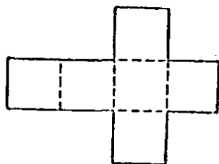
正六面體
