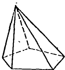
斜角錐
