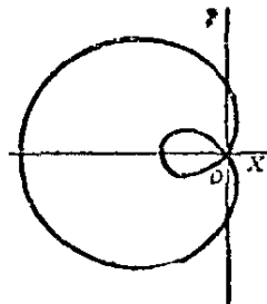
蝸線 LIMACON
