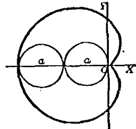
心臟線 CARDIOID
