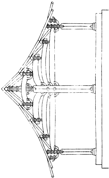
三層分層屋椽
