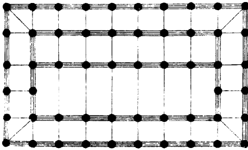
殿間地盤殿身七間副階 周市各兩椽身內單槽
