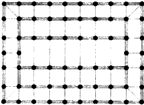
殿間地盤殿身七間副階 周市各兩椽身內雙槽
