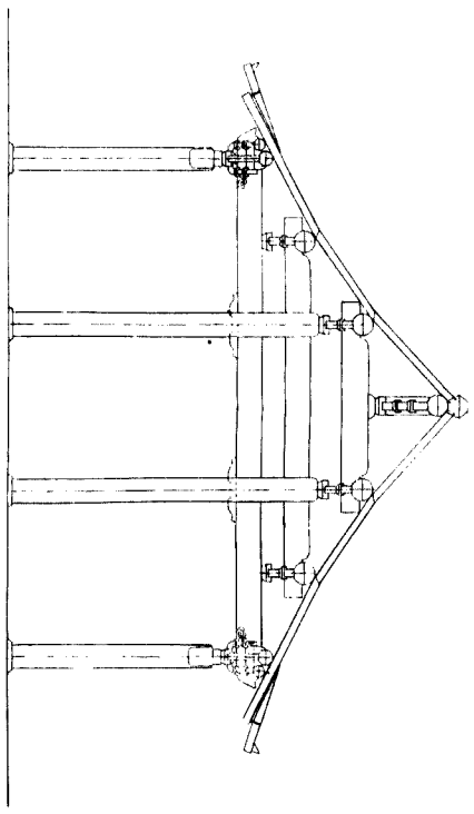
大梁屋架乳栱對四椽椽用柱 七架梁四柱做法同後圖材料三彩
