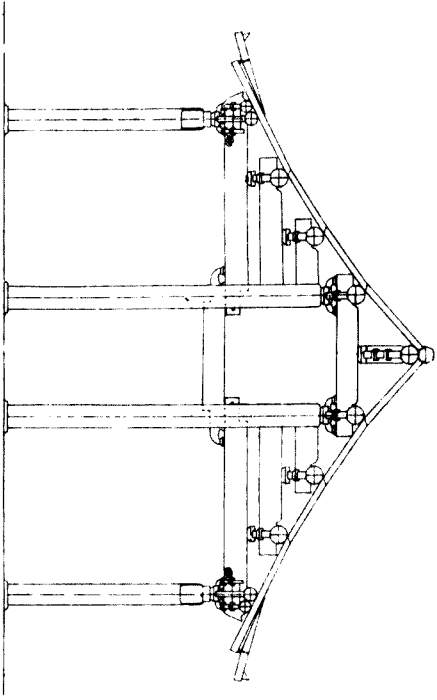
八、椽架前後三椽架用柱 九、椽架前後三椽架用柱 十、椽架前後三椽架用柱 十一、椽架前後三椽架用柱 十二、椽架前後三椽架用柱
