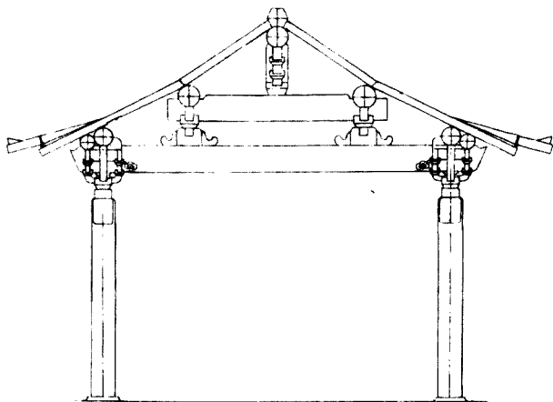
四架椽屋通檐用二柱
