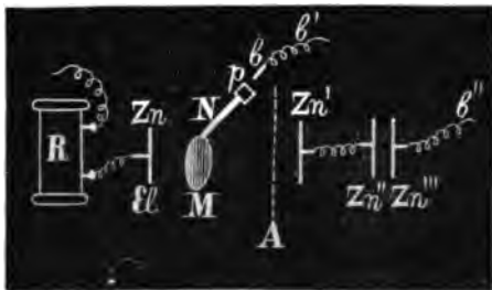
Рис. 19. R—бобина; ZnEl—электродъ; NM—препаратъ; Zn' и Zn''—металлическія пластинки, соединенныя проволокою; Zn'''—такая же большая пластинка, какъ и Zn'', соединена съ землею, служитъ для усиленія дѣйствія пластинки Zn'' (конденсаторъ); bb'—проволока отъ земли.
