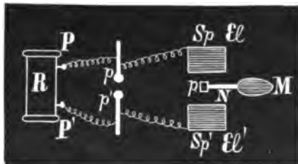
Рис. 32. R—бобина; pp'—разрядникъ; SpEl, Sp'El'—концевыя спирали; pNM—препаратъ.
