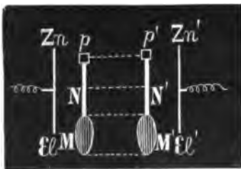
Рис. 36. ZnEl , Zn'El' —электроды; pNM , p'N'M' —два препарата.
