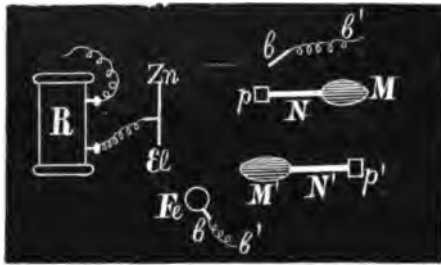
Рис. 18. ZnEl—электродъ; рNM и р'N'M'—лягушечьи препараты въ разныхъ положеніяхъ; bb'—провода отъ земли; Fe—свернутая металлическая пластинка.
