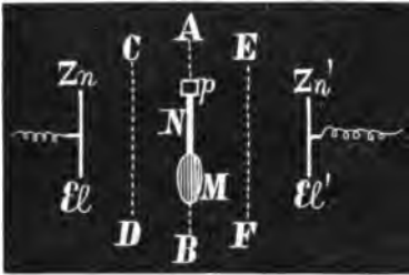
Рис. 31. ZnEl, Zn'El' — электроды; NM — препаратъ въ срединной плоскости АВ.
