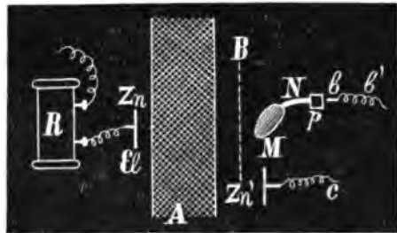
Рис. 17. R—бобина; ZnEl электродъ; А—стѣна; NMр—препаратъ; bb'— проволока отъ земли; Zn'—металлическая пластинка, соединенная проволокою съ электрометромъ.
