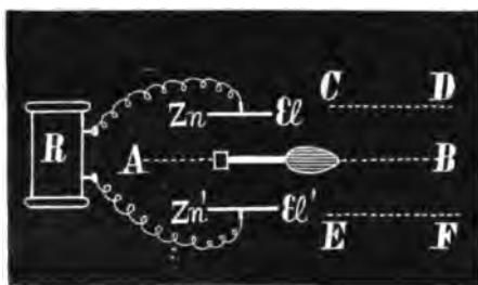
Рис. 30. R—бобина; ZnEI , Zn'EI' —электроды; между ними въ срединной плоскости АВ расположенъ NM-препаратъ.
