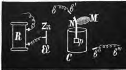
Рис. 20. R—бобина; ZnEl—электродъ; C—полый металлическій цилиндръ; внутри его свѣшивается нервъ; препаратъ укрѣпленъ за косточку; bb' и b''b''' —проводники отъ земли.
