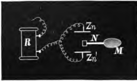
Рис. 12. R —бобина; Zn и Zn' —двѣ пластинки одного и того-же электрода; NM —лягушечій препаратъ между ними (въ разныхъ положеніяхъ: продольномъ, поперечномъ, косомъ).
