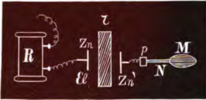
Рис. 9. R—бобина; ZnEl—электродъ; г—парафинъ или стекло; Zn'—металлическая пластинка; NM—глушецъй препаратъ.
