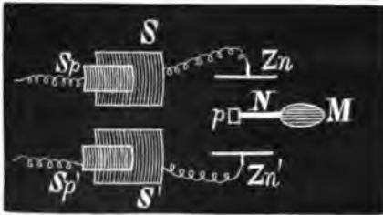
Рис. 33. S, S' —большія катушки вокруг концевыхъ спиралей Sp и Sp' (ср. рис. 31); Zn, Zn' —электроды; pNM —препаратъ.
