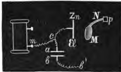
Рис. 2. R—бобина; m—боръ; ZnEl—электродная пластинка; a—побочная пластинка; bb'— проволока отъ земли съ концевой пластинкою.
