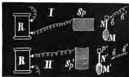
Рис. 23. R—бобина; Sp, Sp'—концевыя спирали, служащія электродами; NM, NM'—препараты; bb'—провода отъ земли
