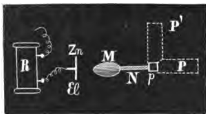
Рис. 8. R—бобина; ZnEl—электроды; NM—лягушечій препаратъ; PP'—„хвостъ“ изъ мокрой бумаги въ продольномъ или поперечномъ положеніи.
