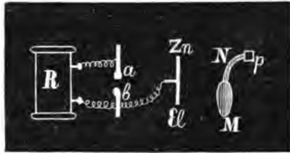
Рис. 1. R—бобина Ruhmkorff'a; ab—разрядникъ; ZnEl пластинчатый электродъ; NM—нервно-мышечный препаратъ; p—кусокъ позвоночника.
