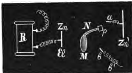
Рис. 3. R—бобина; ZnEl—электродъ-возбудитель; NM—нервъ съ мускуломъ; Zn'—большой конденсаторъ; bb'—проволока отъ земли.
