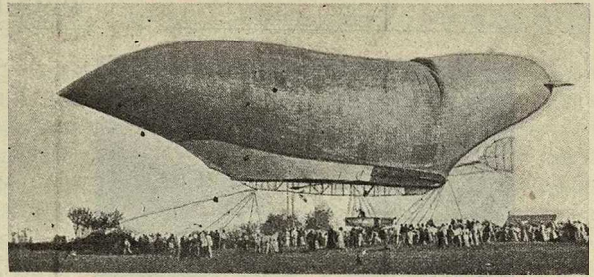
Дирижабль „Республика“ спускается около Преси.
