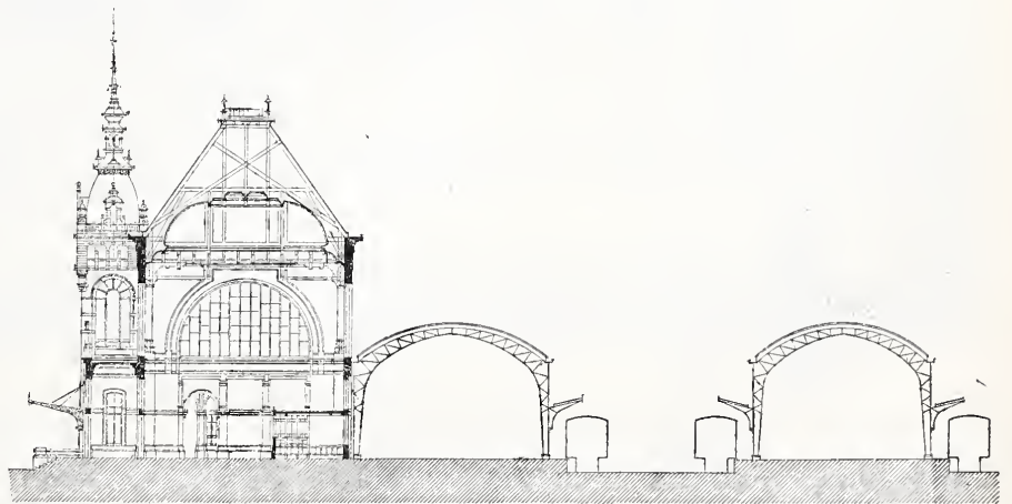
Doorsnede over de Vestibule.
