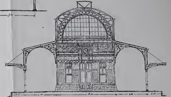
VORRAANZICHT
