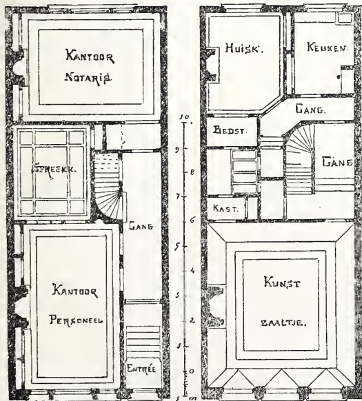
Bel-étage.
