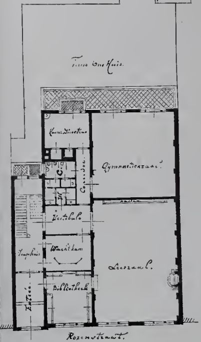
BEGANE GROND
