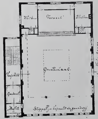
TWEDE VERDIEPING
