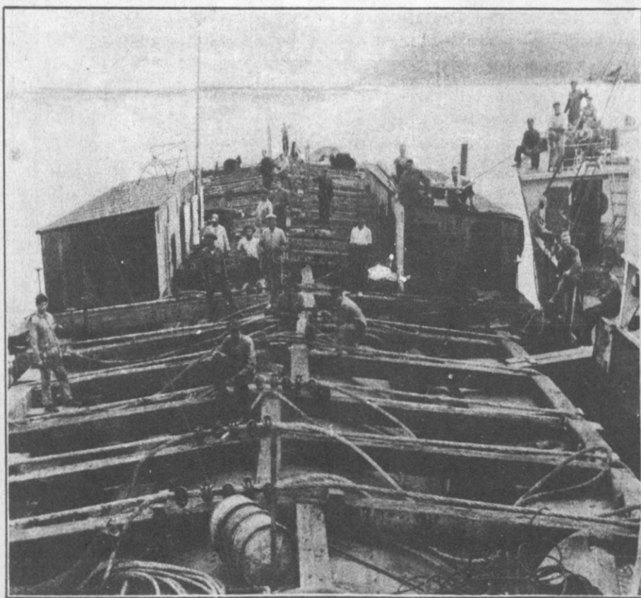
Dok, pripravljen za dviganje potopljene ladje, ki leži 50 m pod vodno gladino.
