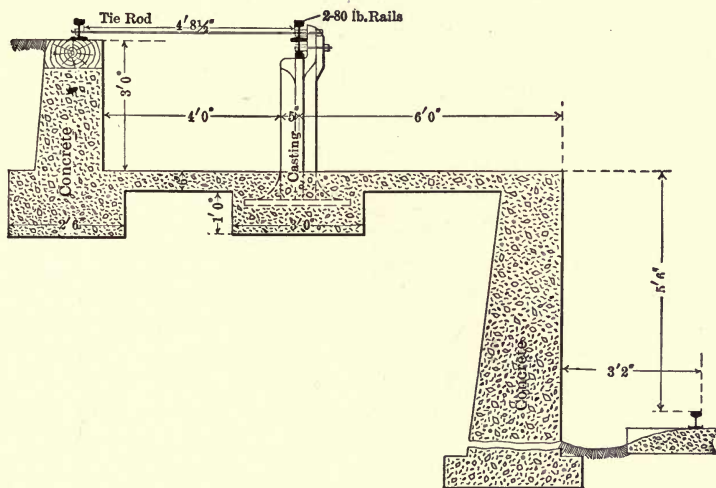
Fig. 77. Depressed Ash Pit.
