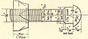
Fig. 3. Harvey Grip Bolt.
