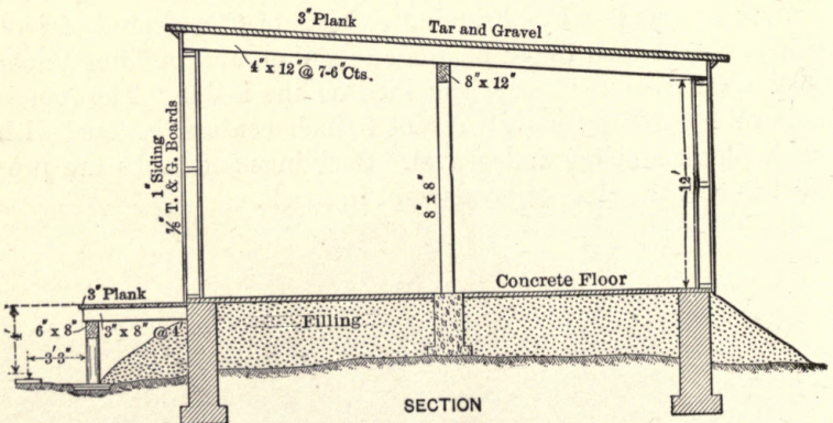
Fig. 62. Storehouse.
