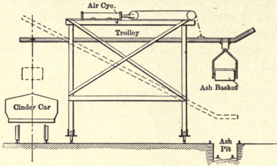
Fig. 78. Gantry Crane.
