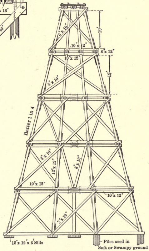
Fig. 30a. Frame Trestle.
