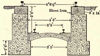
Fig. 75. Deep Ash Pit.
