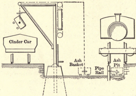
Fig. 79. Ord Ash Pit.
