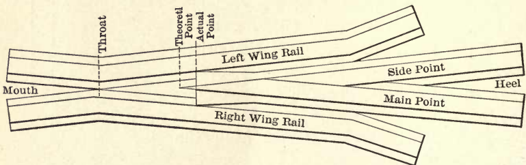
Fig. 7. Rigid Frog.
