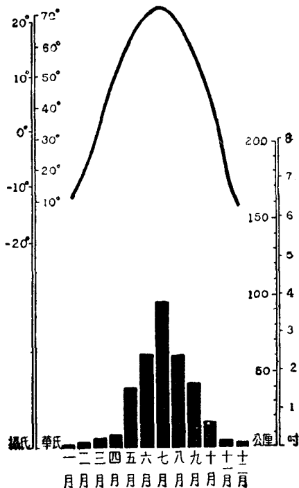
內蒙古的氣候狀況 基於西灣子(338公厘)與二十四頃地(335公厘)之紀錄。
