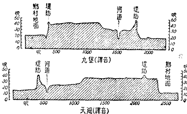
黃河河床及其鄰近地區的橫剖面
