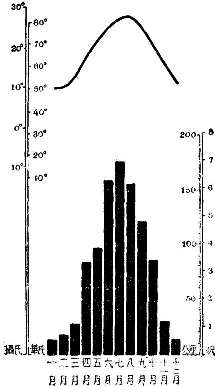
紅色盆地的氣候狀況 雨量記號表基於重慶 (1,103 公厘)，成都 (880 公厘) 安岳 939 公厘)。溫度亦同。
