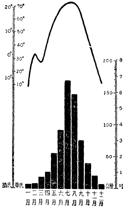
東北平原的氣候狀況 雨量依據營口 (639公厘)、瀋陽 (672公厘)、公主嶺 (618公厘)、哈爾濱 (537公厘)等處資料計算。溫度亦同(公主嶺除外)。
