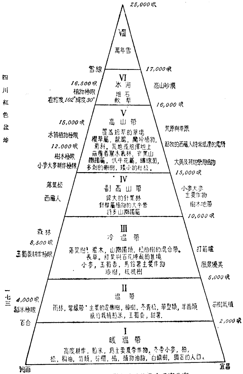
四川盆地與康藏山地植物帶之垂直分布 依據 E. H. Wilson, [A Naturalist in Western China] Courtesy Methuen and Co.
