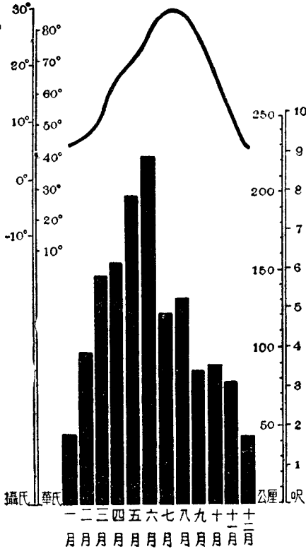
長江平原的氣候狀況
