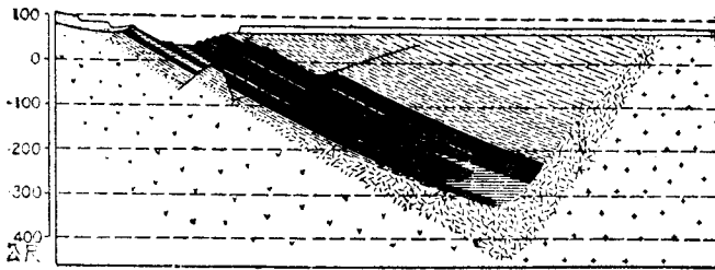
撫順煤層的剖面
