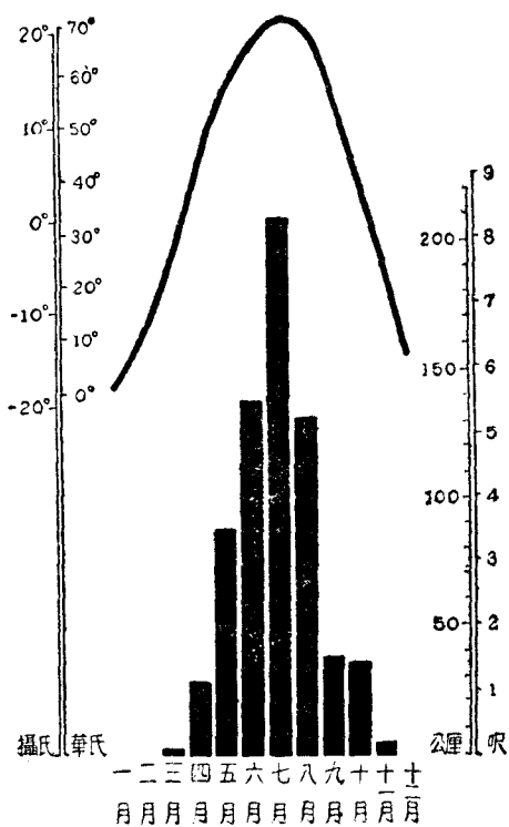
長白山地的氣候狀況
