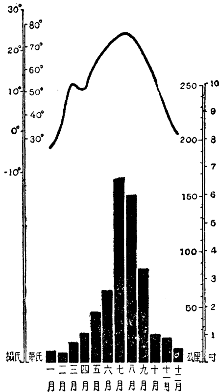
環黃渤海山地之氣候狀況
