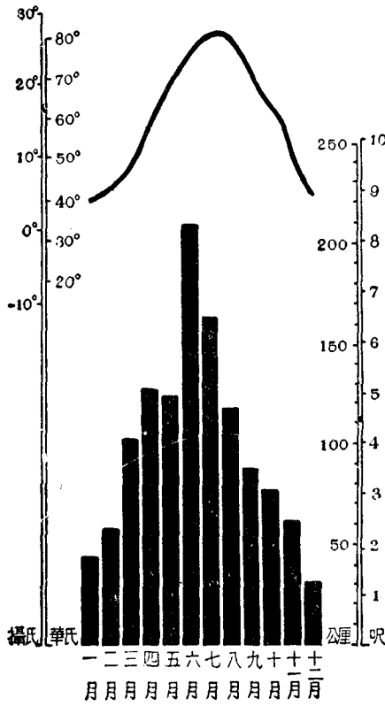
江南丘陵的氣候狀況 根據長沙的雨量(1,412公厘)
