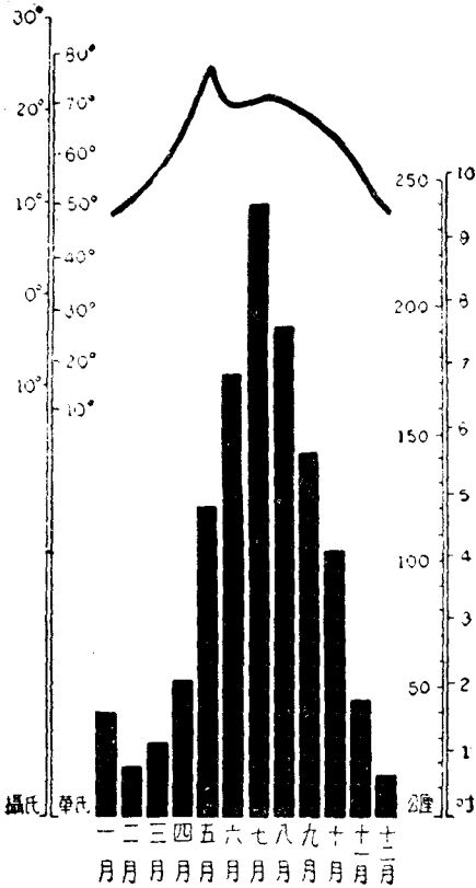
西南高原的氣候狀況
