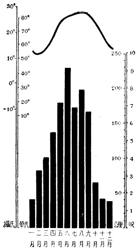
東南沿海山地的氣候
