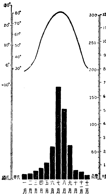
華北平原的氣候
