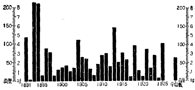
天津六月降雨量
