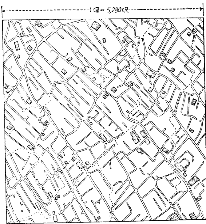
三角洲地方(上海東南方)一方哩的運河水系 運河間的平均距離為 380呎。河道大部輻屬可航。 小徑用點線，農莊用小方塊斜線以表示之。
