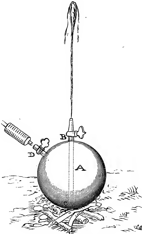
FIG. 5.—De Caus's Apparatus, A. D. 1605.
