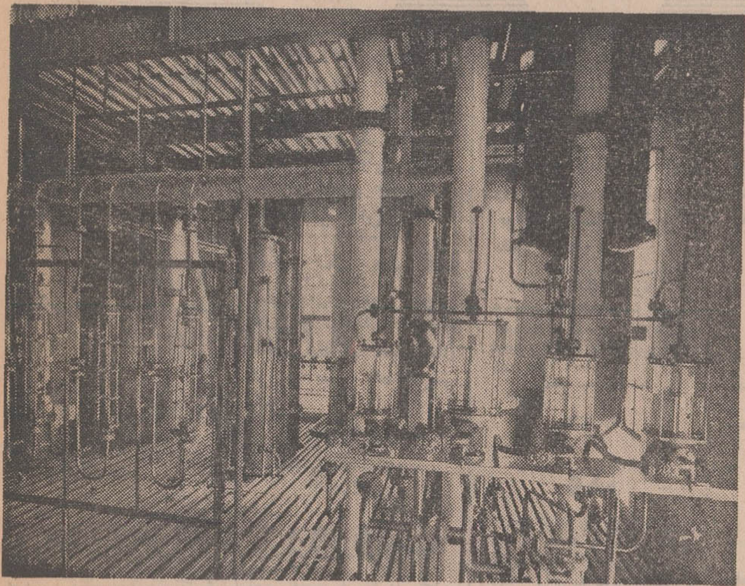
قسمتی از دستگاه تقطیر الکل کارخانجات ایران می اهواز
