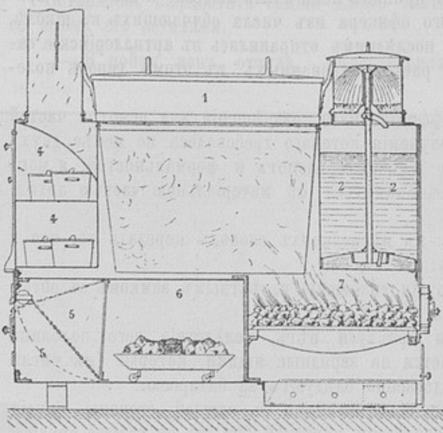
1) Котель для продуктовъ. — 2) Кофейникъ. — 3) Горячая вода. — 4) Согрѣваніе котелковъ должностныхъ. — Помѣщеніе для готовой пищи. — 6) Печь. — 7) Топка. — 8) Подъемная полка. — 9) Дверцы въ помѣщенія (4). — 10) Дверцы въ помѣщенія (5) и (6).
