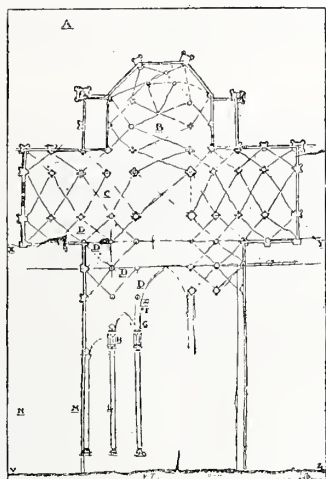
PIANTA DEL DUOMO
