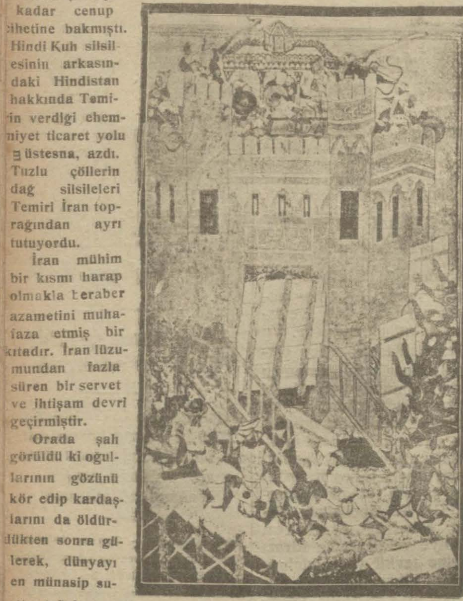
Tatar ordusu bir şehir kapısına hücum ediyor
