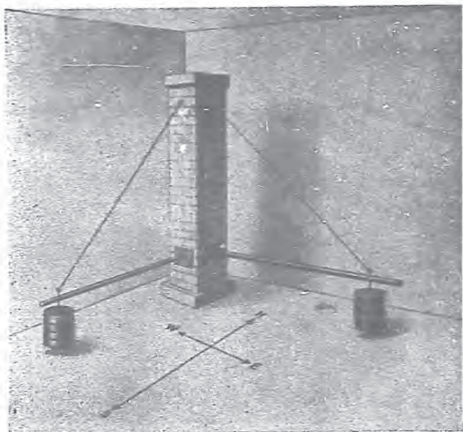
圖三 地震記錄器的要點。地球的任何振動傳到磚的稜錐體，使二柄作微細角度的搖擺。這些搖擺由機械的槓杆擴大，而加以記錄，如下圖。
