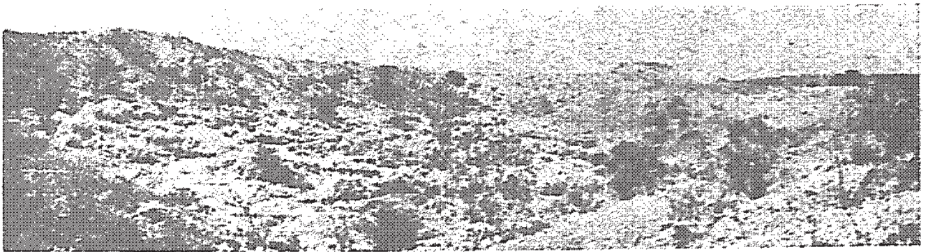
圖四十九 另一景示全上陷口的內部。
