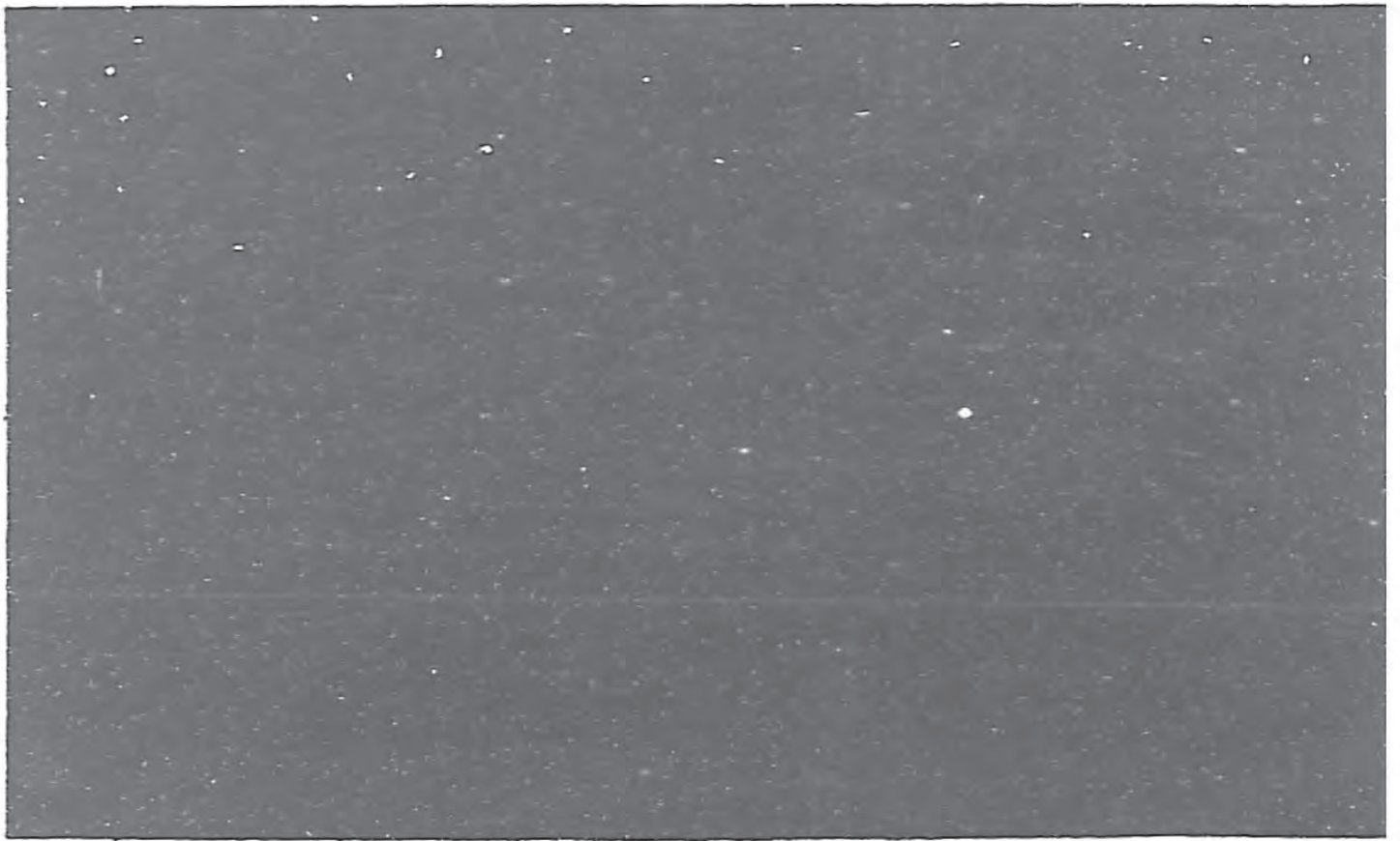
圖九十四 全前(圖九三)的星野,展露至二十等的恆星。
