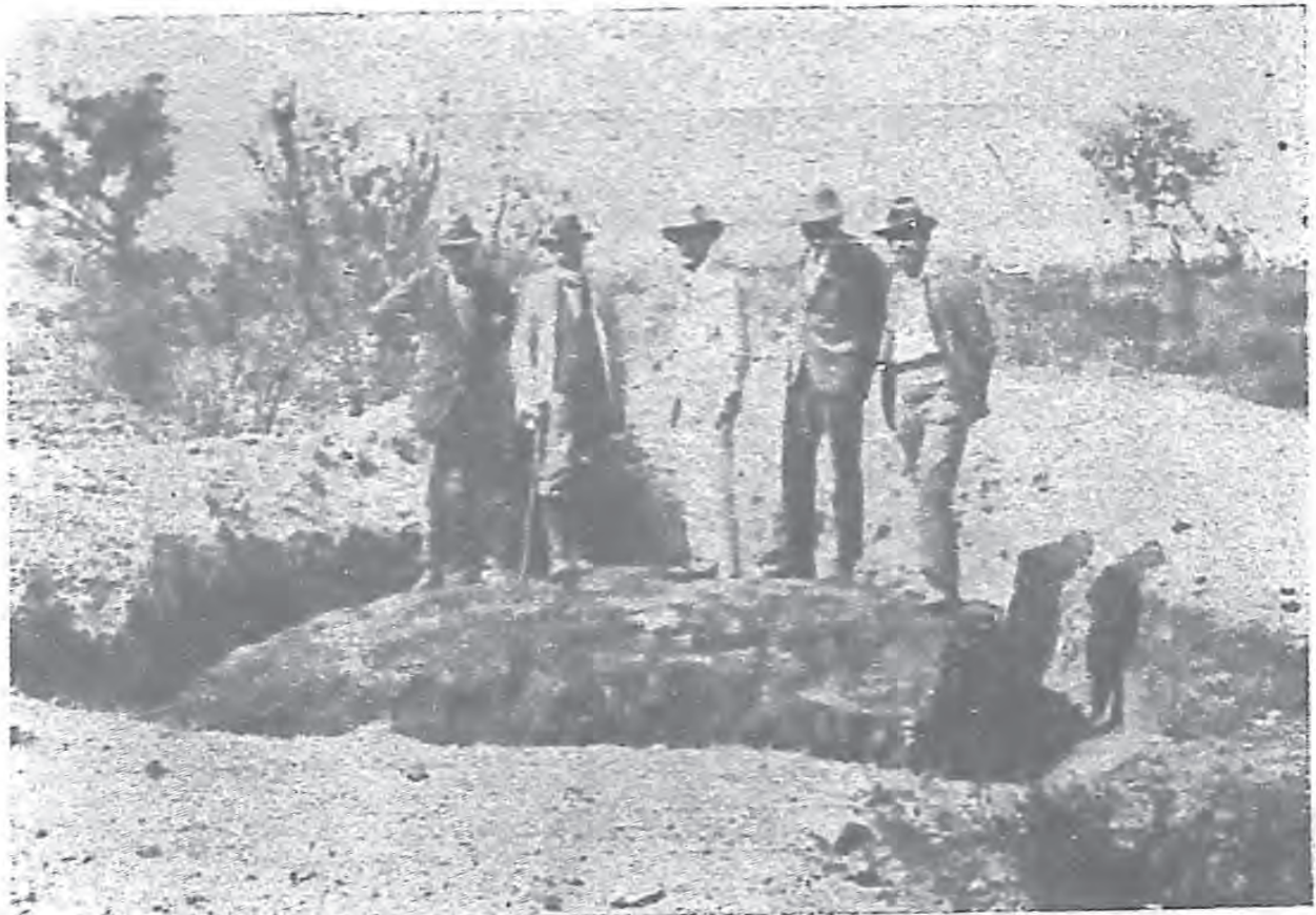
圖四十四 巨大的 荷巴 (Hoba)隕石,估重六十噸。
