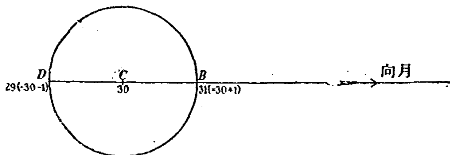
圖六十八 月對地所施潮汐力之圖解
