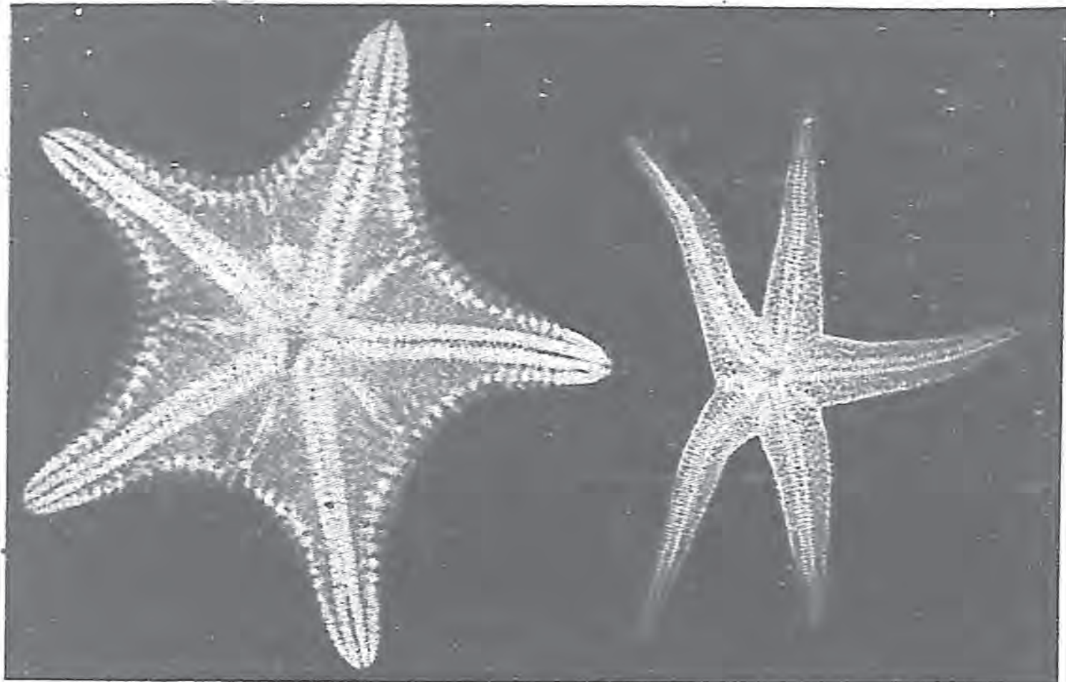
圖九十 用X-輻射所見的星魚
