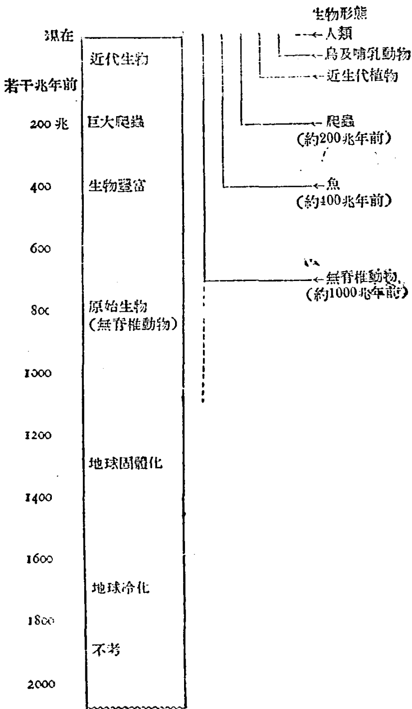
圖二十八 地球古史的主要時期及大事表 (事情和年代概屬推測的)
