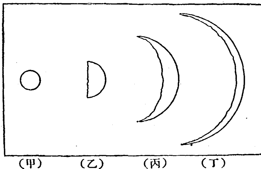
圖四十三 金星的相(盈虧)：(甲)離地球最遠時——正圓形，直徑 9\frac{1}{2} 秒；(乙)在天空中離日最遠時——半圓形，直徑18秒；(丙)最明朗時——一彎眉，直徑40秒；(丁)在可見到的直徑最大時——一彎眉，直徑62秒。
