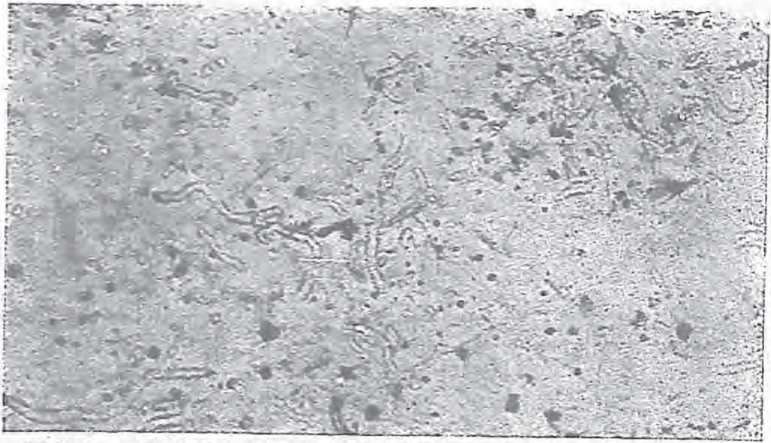
圖十五 已知的最古化石——極微藻類。照片所示一薄片岩石切得很薄，可以透明。此約放大一百九十倍。
