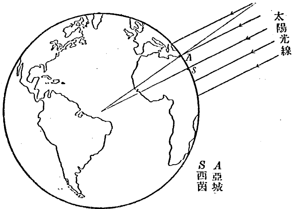
圖一 埃拉托色尼 發見太陽光線垂直射在 西茵 時，與 亞城 的垂直點相距為一全圓之五十分之一。他得到結論：地球的圓周是五十倍於 亞城 與 西茵 的距離。
