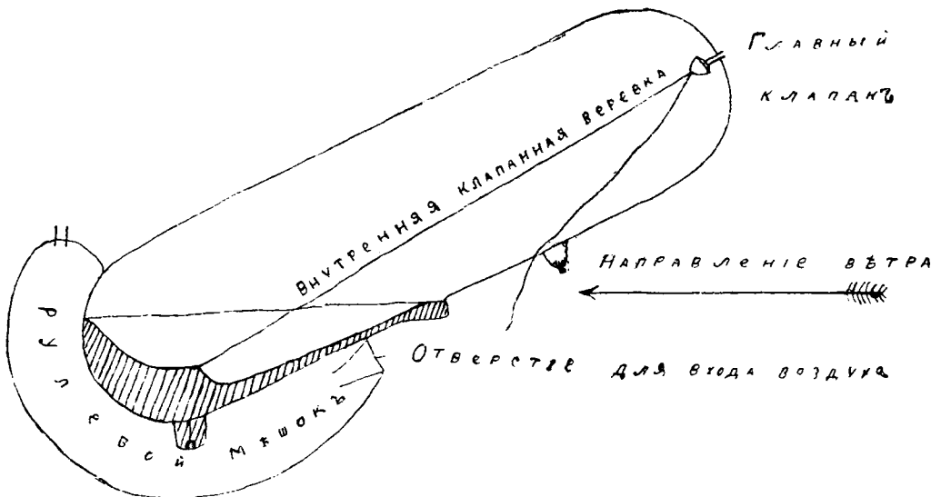
Чертежъ № 2.
