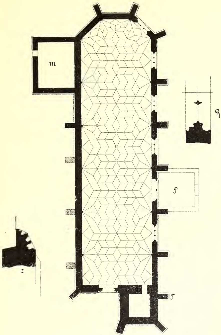
A templom alaprajzának léptéke 10 m
