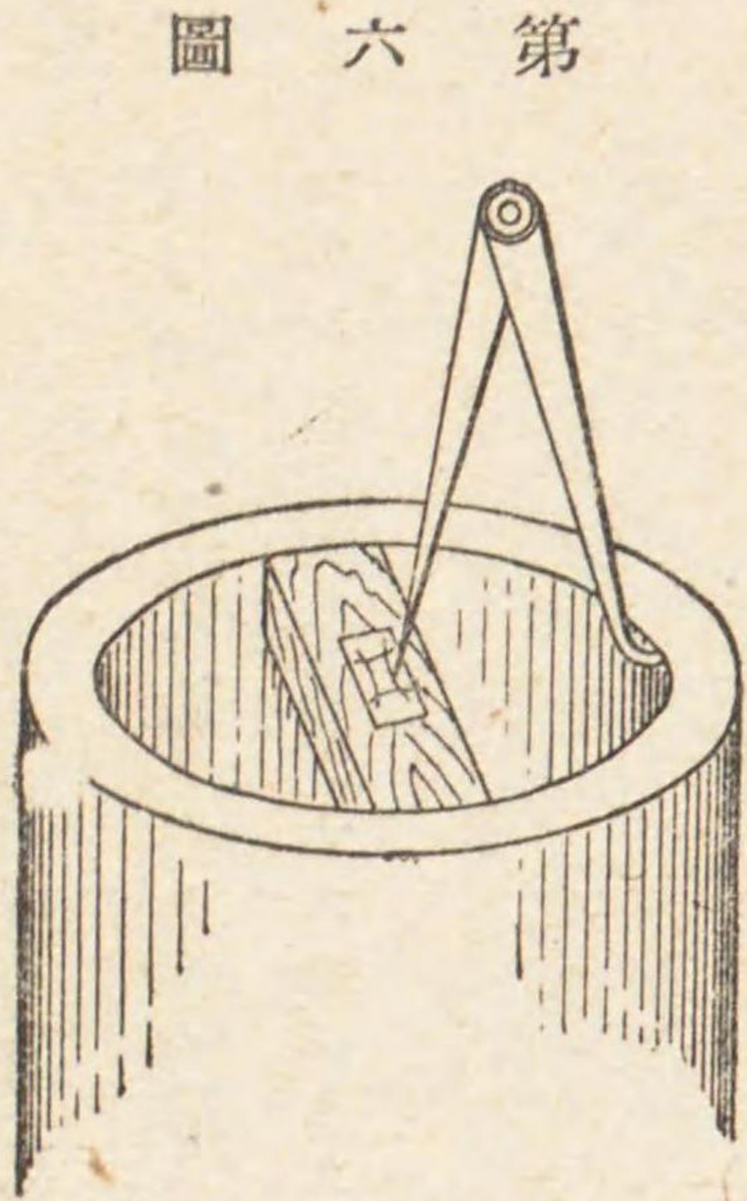
第三十九 第六圖ノ如ク孔ニ木片ヲ打チコミ其ノ中央ニ「ブリキ」板ヲ張ルカ又ハ鉛、銅片ニ打チ延バシ其ノ長サヲ孔徑ヨリモ約一〇耗長クシ之ヲ孔ニ打チ込ミテ丸棒ノ場合ト同一要領ニ依リ中心ヲ求ム
