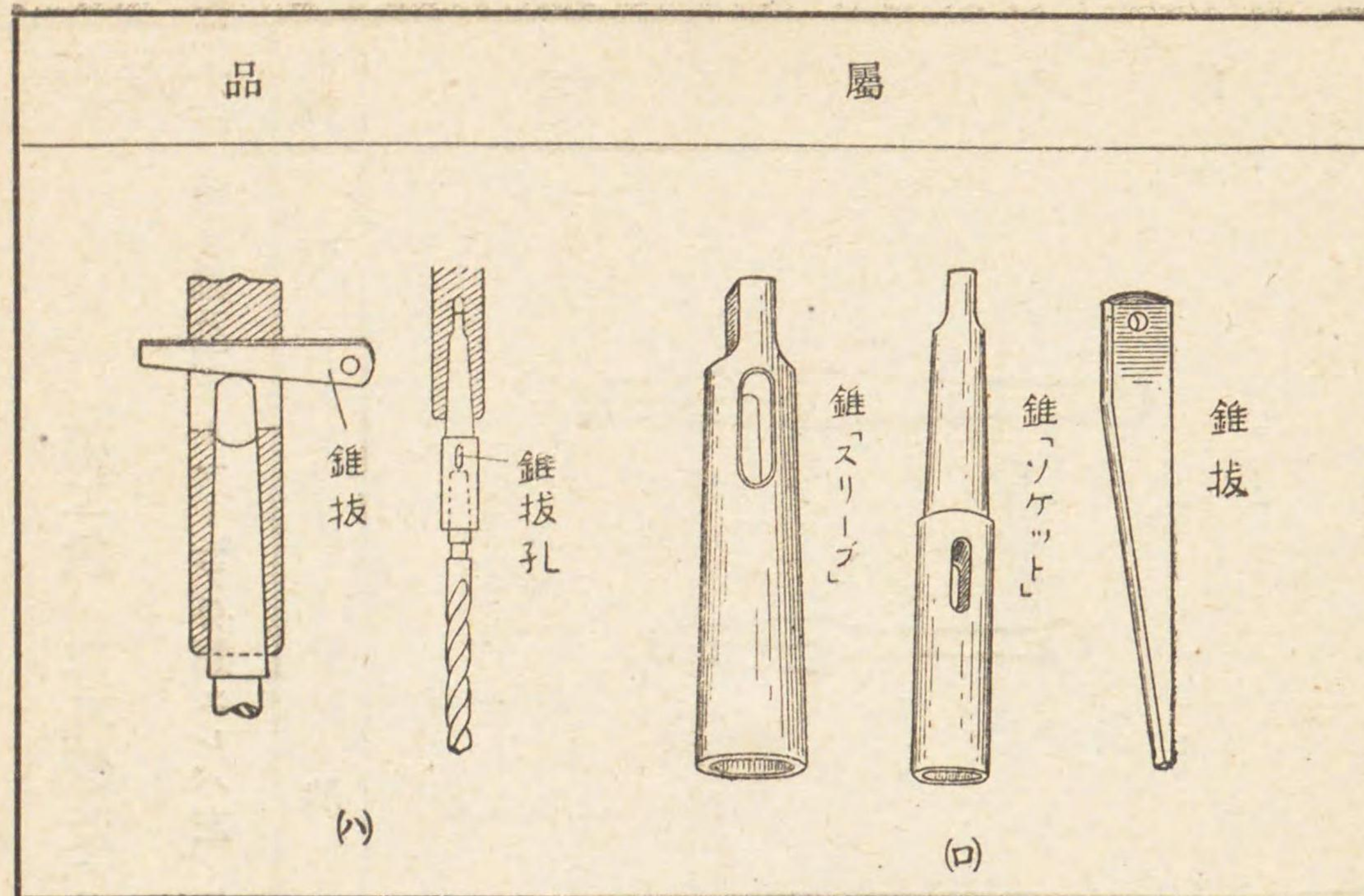
(イ)、(ロ)、(ハ)圖ハ電氣錐屬品ノ一例ヲ示ス
