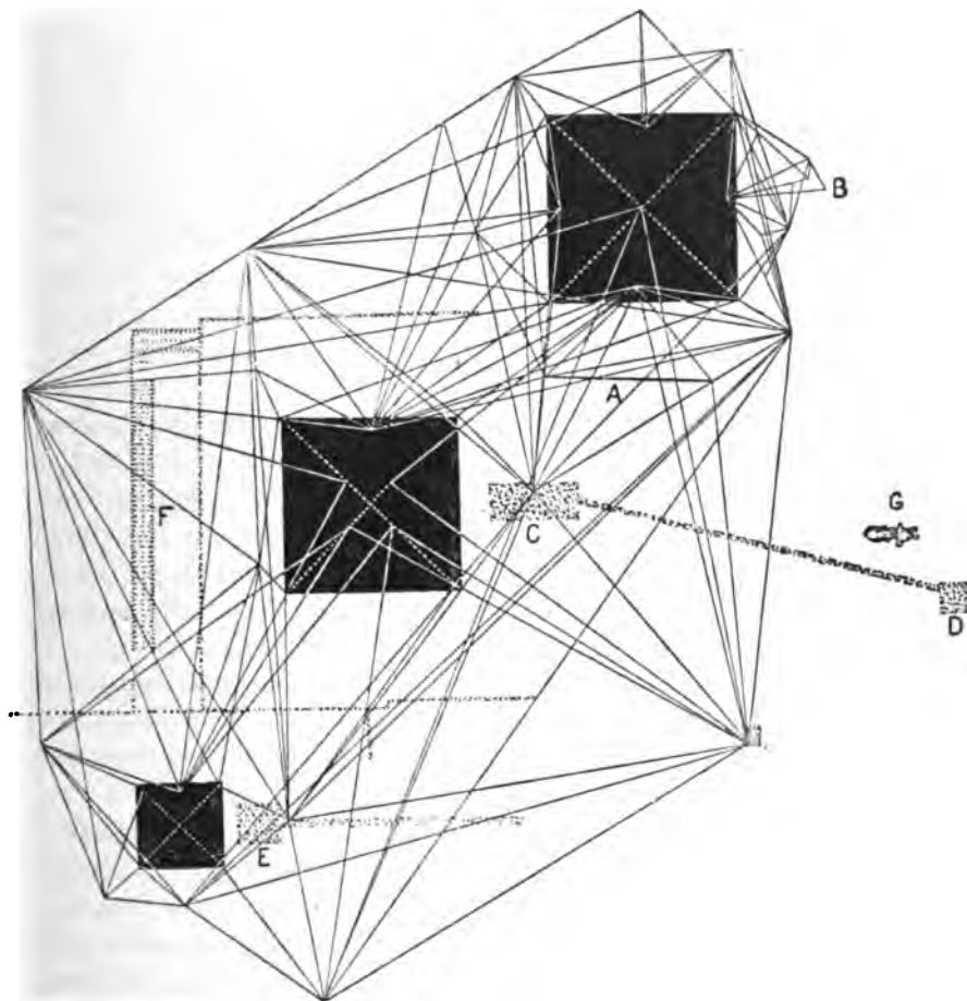
№ 142. Триангуляция пирамидъ въ Гизе.
