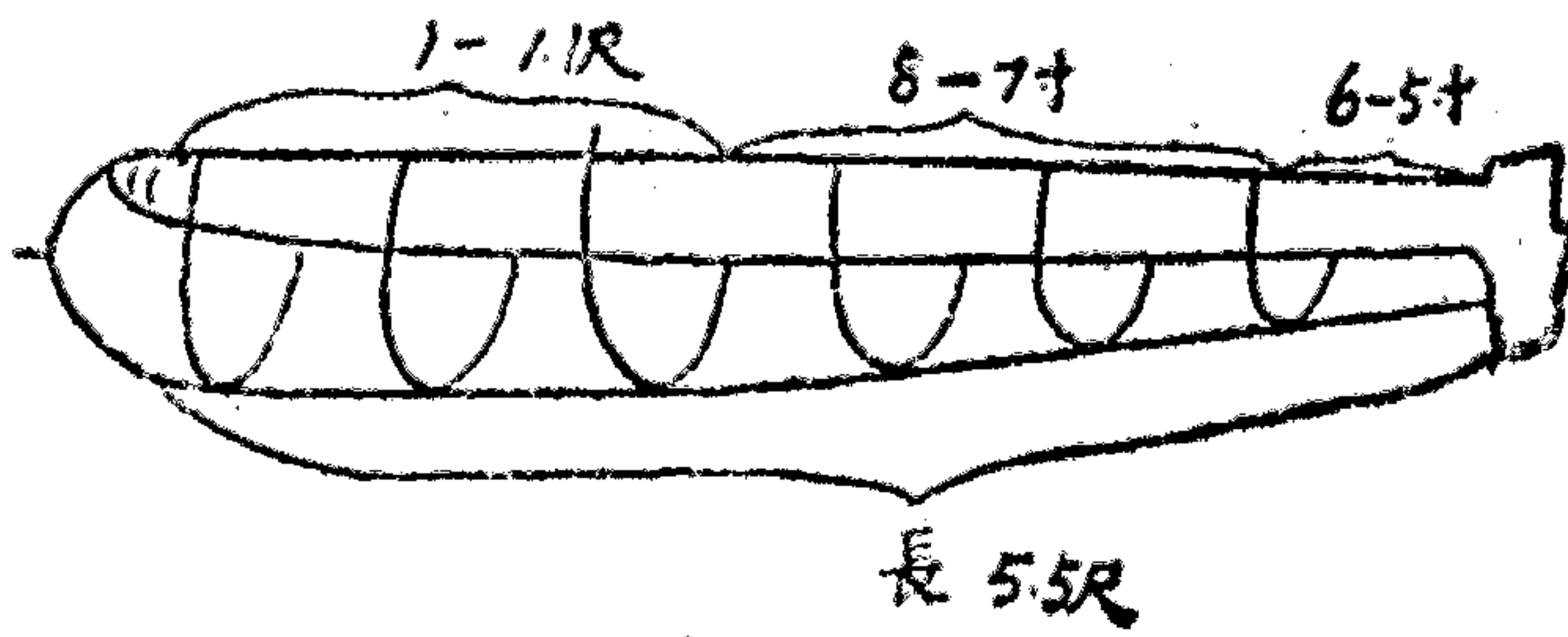
(B) 機身
