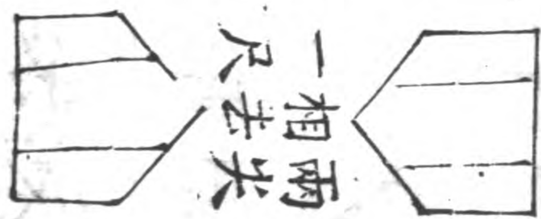
梁口
