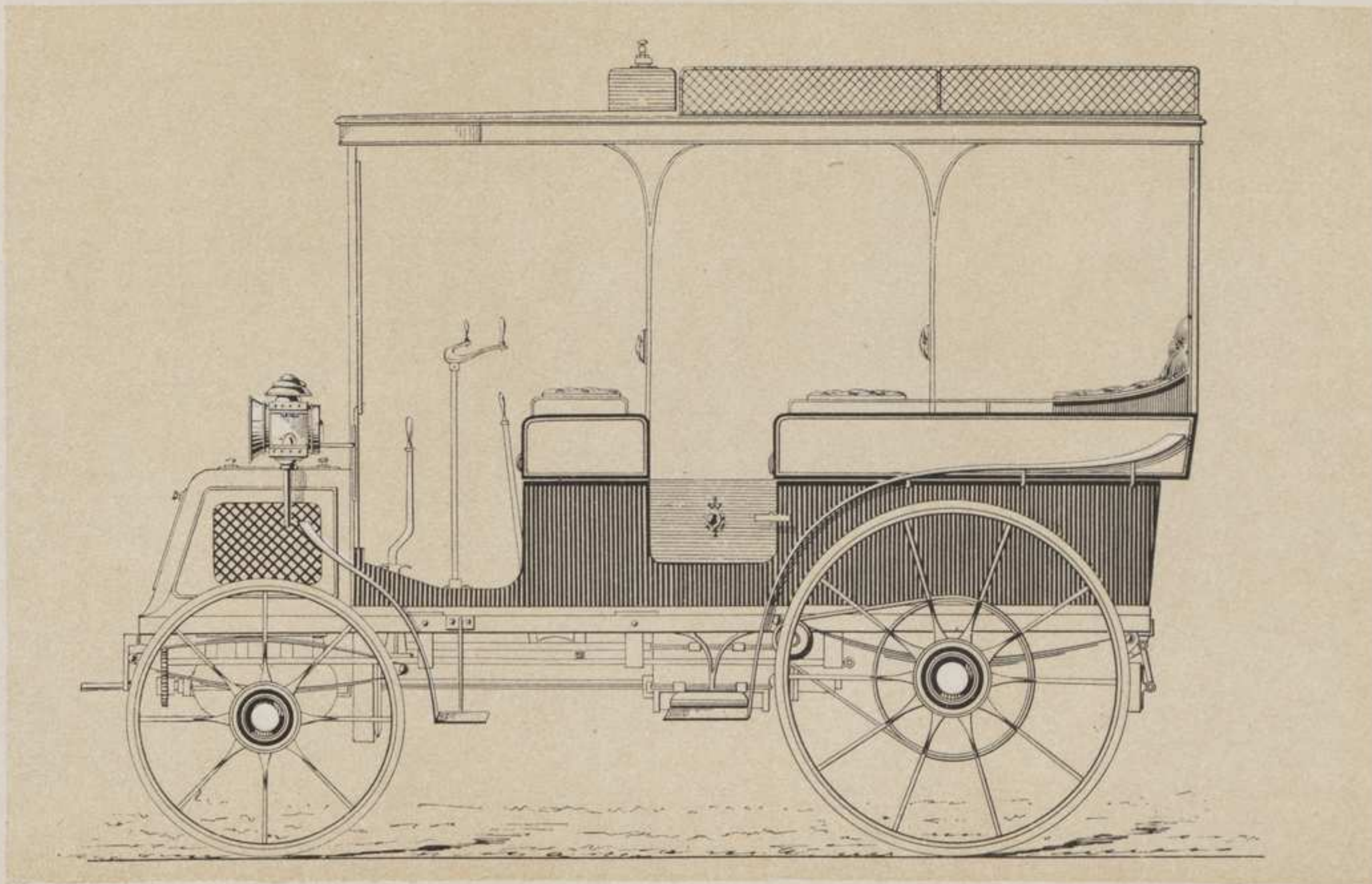
N° 36. — BREAK A 3 SIÈGES PARALLÈLES
