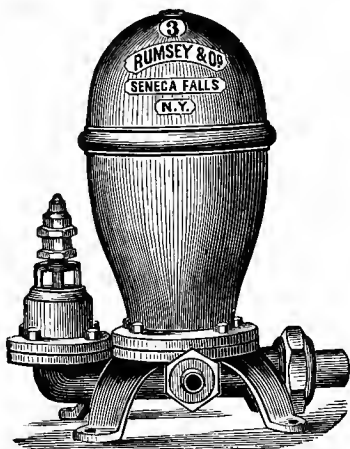
Fig. 77. A standard ram.
