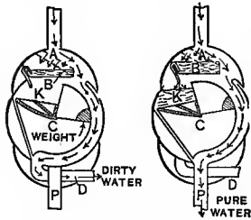
Fig. 21. Rain-water separator.
