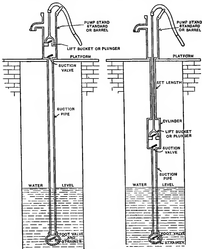
Fig. 30. Lift pumps.
