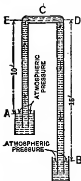
Fig. 57. The siphon.
