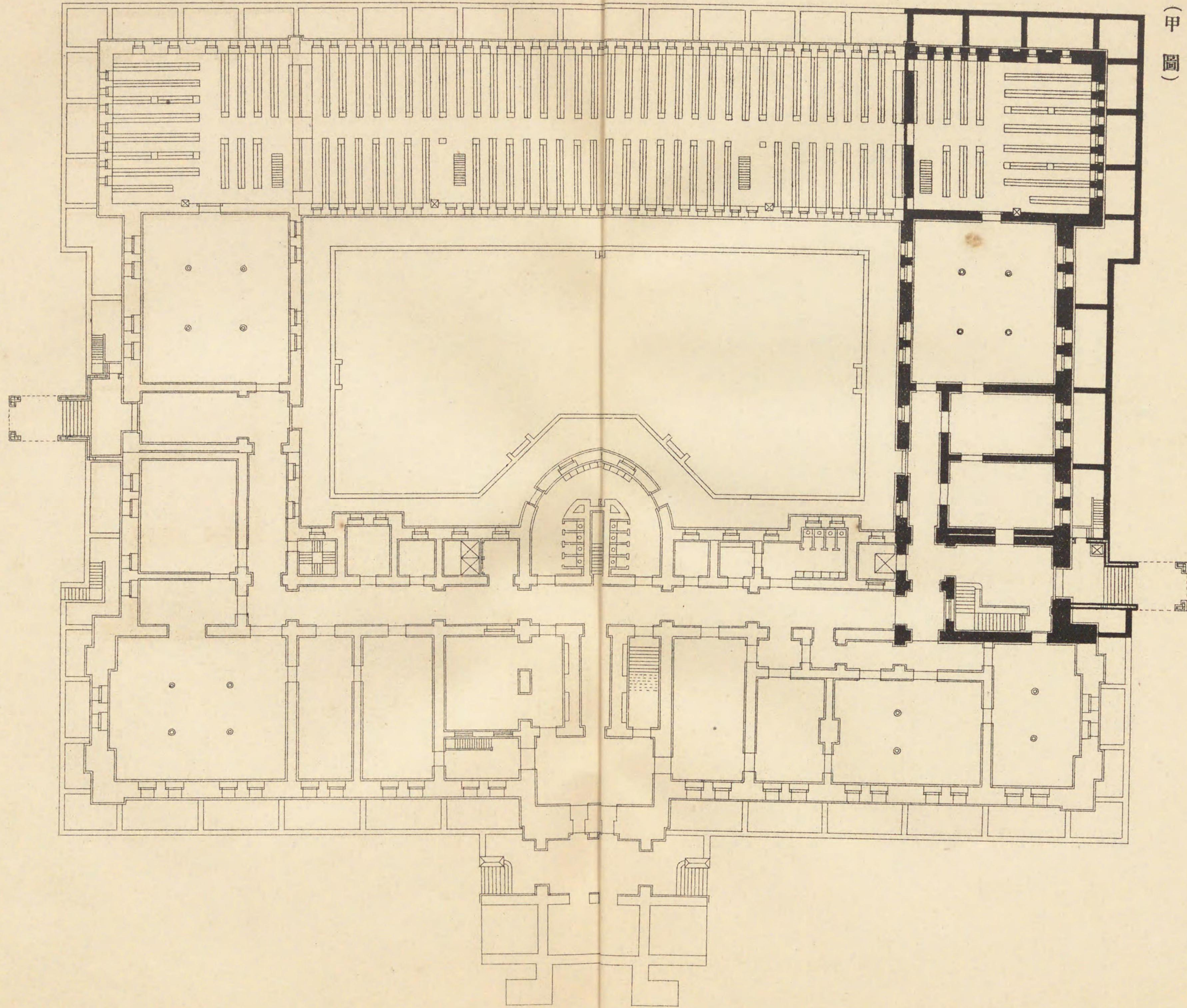
全設計平面圖 (黑色ハ既成部)
