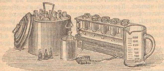
Аппаратъ Сокслета.
