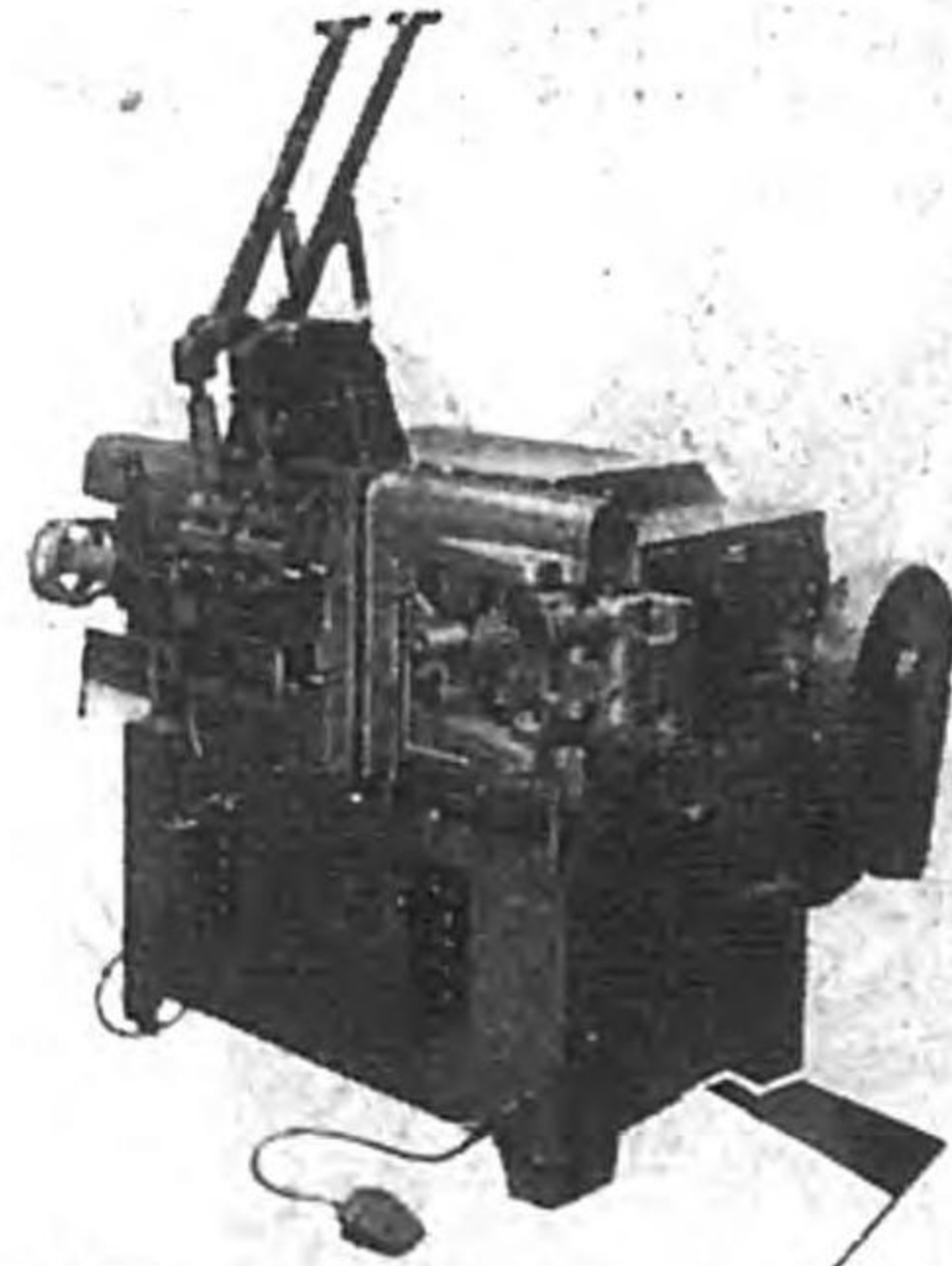
BLM型フラッシュバット溶接器 150KVA
