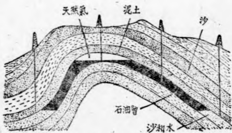
圖一：石油帶位置的縱剖面
