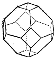
第十五圖 八面體和六面體的聚形
