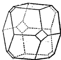
第十六圖 斜方十二面體和六面體的聚形
