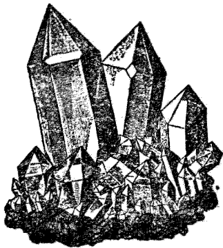
第四十二圖 晶簇
