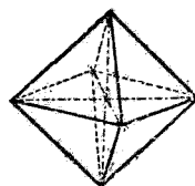
第八圖 八面體
