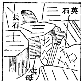
第九十一圖 全晶質組織
