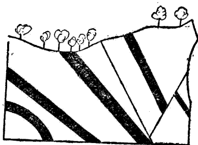
第 八 十 八 圖 煤 層
