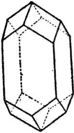
第二十七圖 正方錐和正 方柱的聚形
