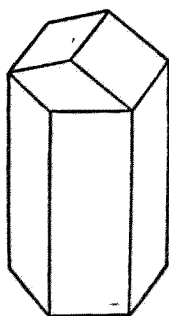
第七十六圖 角閃石晶形
