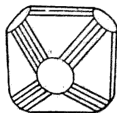
第六十三圖 方鉛礦晶形
