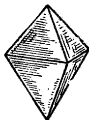
第八十七圖 金剛石晶形
