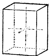
第九圖 六面體
