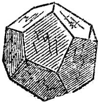
第六十二圖 黃鐵礦結晶
