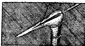
第四十九圖 還原焰
