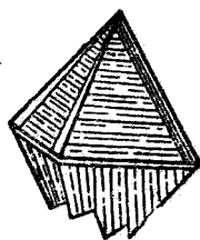
第五十四圖 自然金晶形
