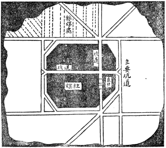
第六圖 長壁法
