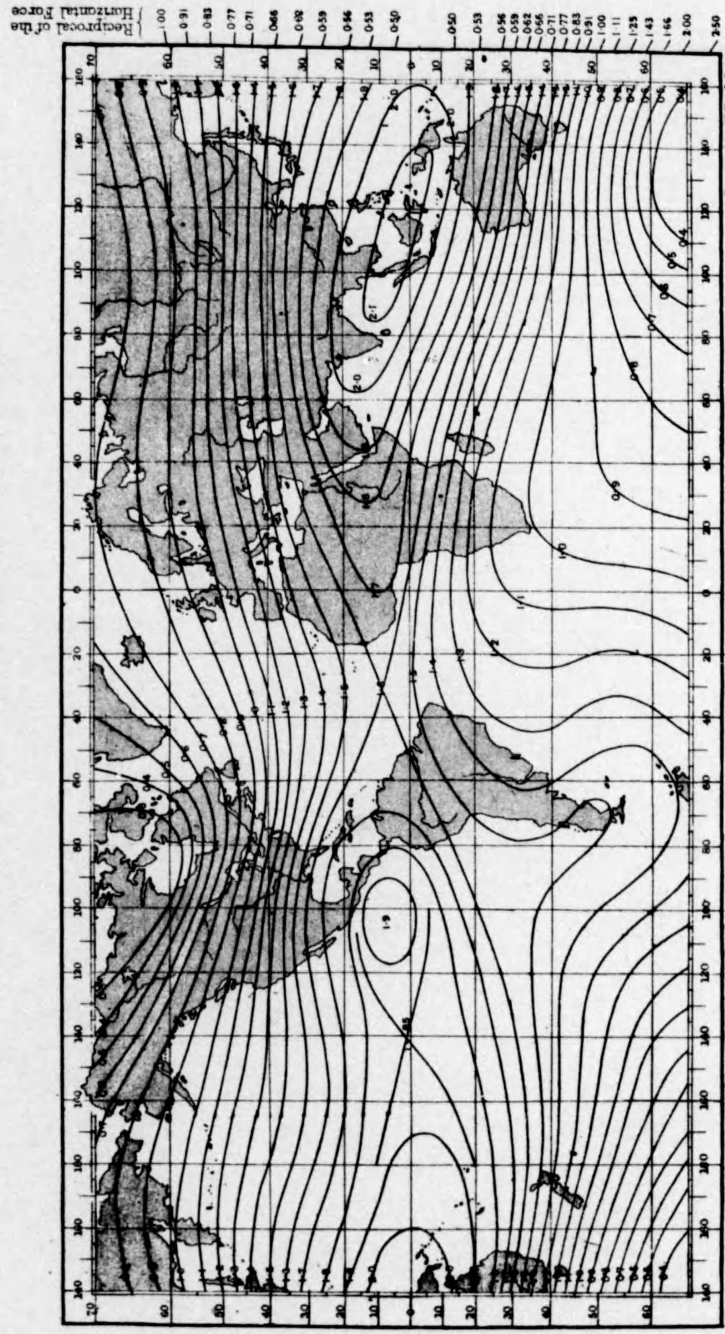
第七十三圖 等水平力線圖 (Lines of equal horizontal force)
