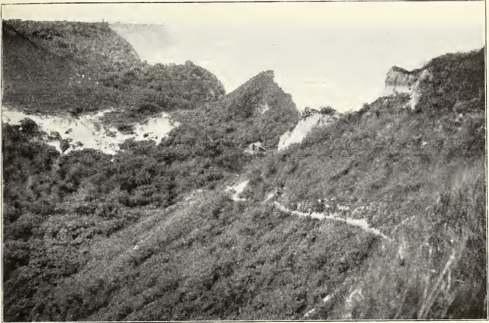
Bild 9. Die westliche Partie der Dirschkeimer Schlucht vom nördlichen Rande aus gesehen. Der Galgenberg, der seewärts steil abfällt, dacht sich nach dem Lande zu unter einem Winkel von ca. 45^{\circ} ab. Aufgen. am 20. VII. 1909.
