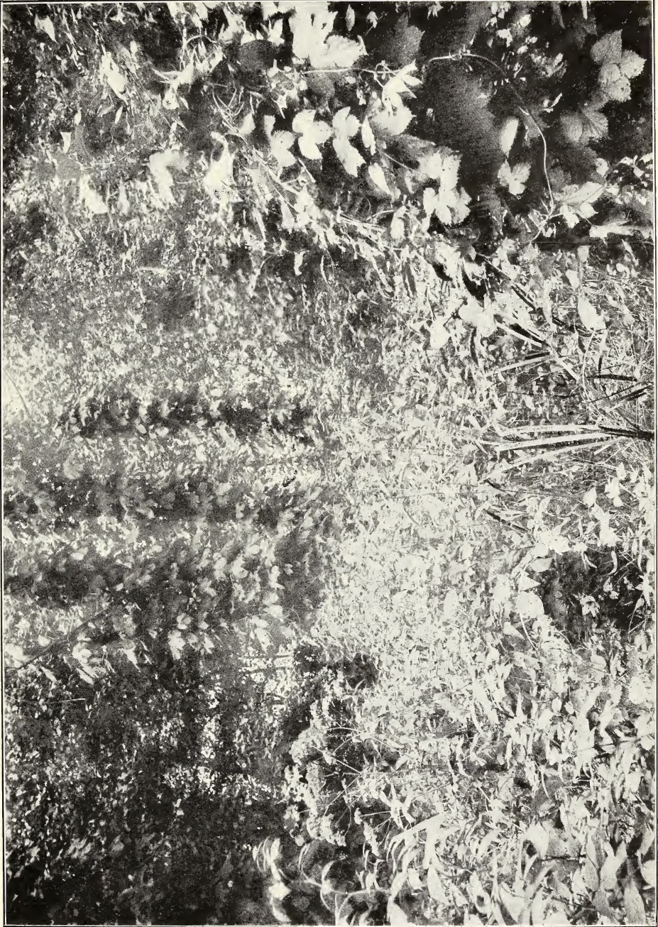
Abb. 3. Erlenstandmoor (in der Nähe des Philippssteiches bei Königsberg).
