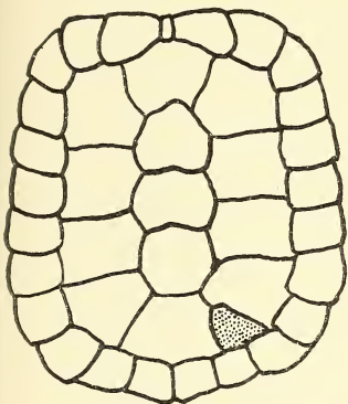
Fig. 3. Testudo graeca . \frac{2}{3} der nat. Größe.
