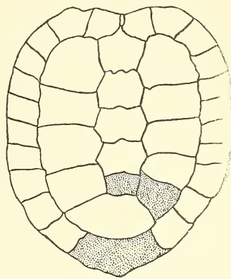
Fig. 5. Testudo graeca . \frac{1}{3} der nat. Größe.
