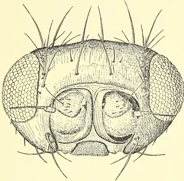
Fig. 3. Carnus hemapterus ♂. Kopf von vorn. Vergr. 162:1.
