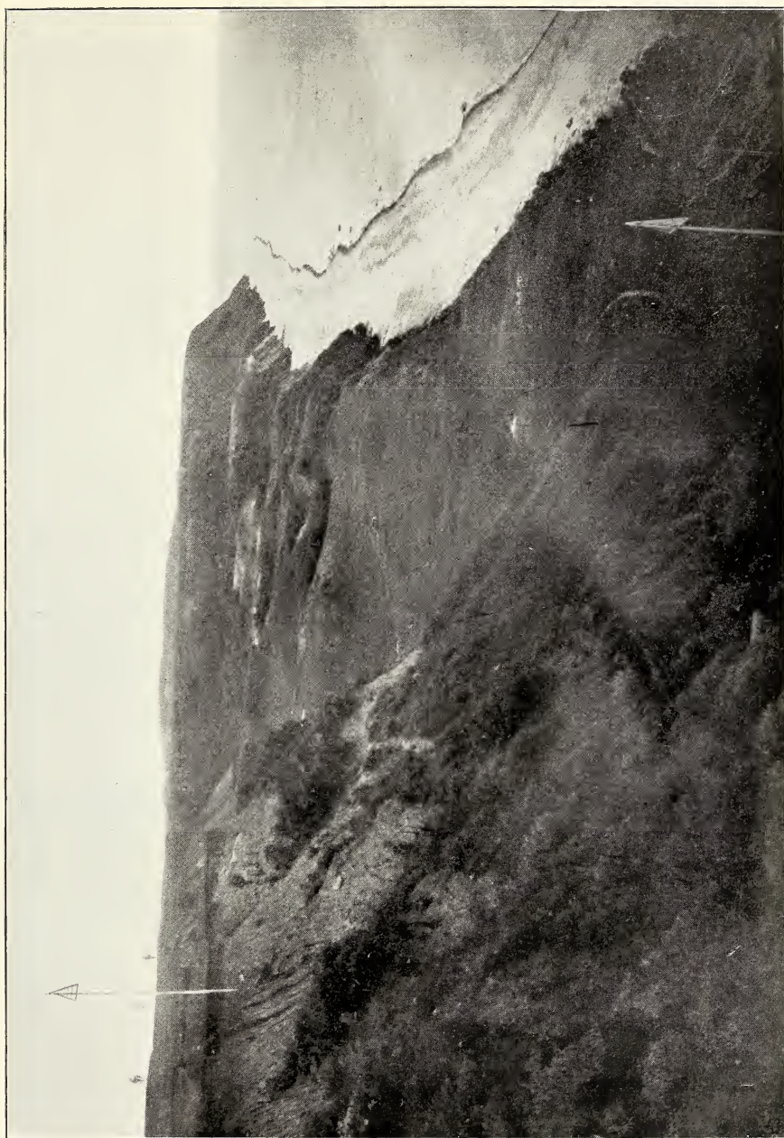
Die Rosenorter Schlucht. Im Hintergrunde die Dirschkeimer Plantage, hinten rechts die Kadlickecke, im Vordergrund die beiden Baken der westlichen Ansteuerungslinie. Aufgenommen am 17. Juli 1912.
