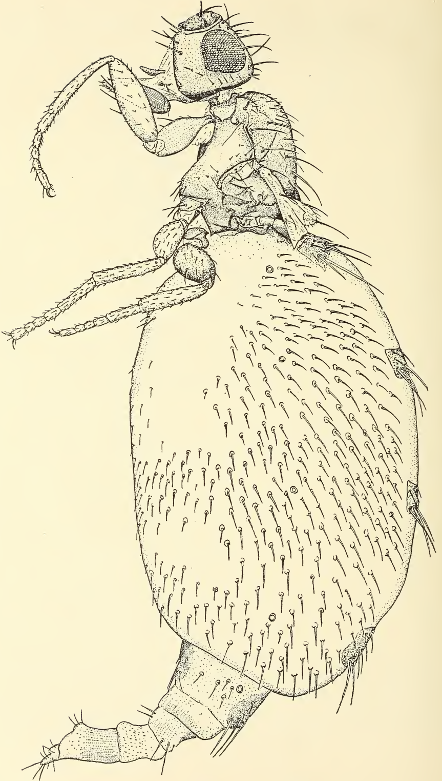
Fig. 2. Carnus hemapterus ♀. Vergr. 60:1.
