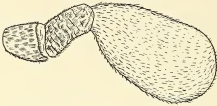
Fig. 7. Carnus hemapterus . Schwinger. Vergr. 250:1.
