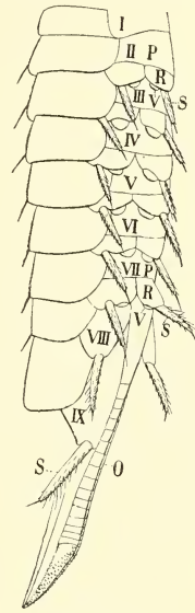
Fig. VI. Lepidothrix pilifera MENGE,
