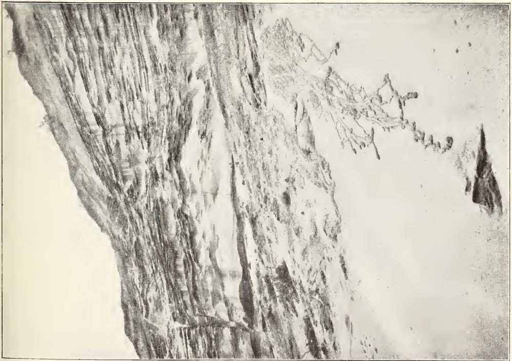
Bild 5. Der Dirschkeimer Sand vom Winde in seinen festeren Partien herausgearbeitet. Links oben eine Erosionsrinne, rechts unten Tongerinne auf der Sandböschung. Aufgen. am 31. VII. 1909.
