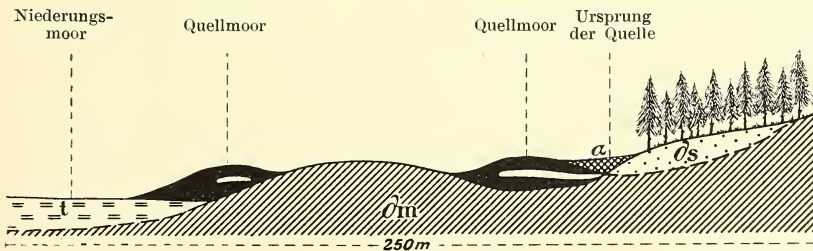
Abb. 1. Quellmoore auf der Gr. Bodschwingker Wiese unmittelbar am Pillwung-See (Kr. Oletzko).
