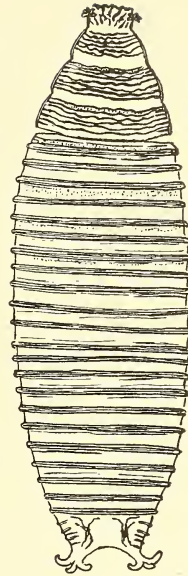
Fig. 11. Carnus hemapterus . Puparium. Vergr. 40 : 1
