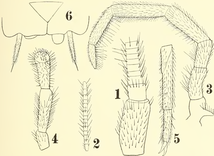
Fig. XIV. Praemachilis cineracea (v. OLF.).
