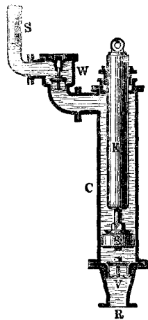
Насосъ Рнс. 1.
