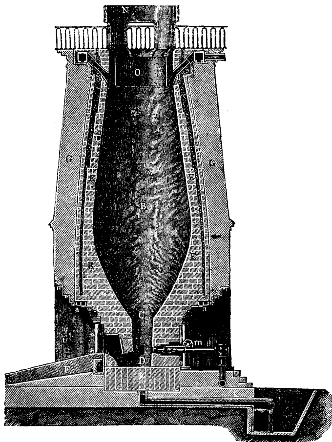
Доменная печь.
