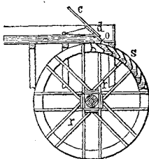
Наливное колесо.
