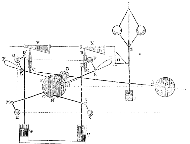
Схема парораспределительнаго механизма Корлиса.
