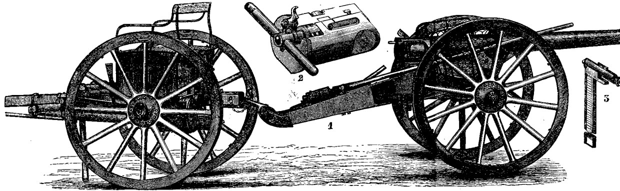
1) Полевая пушка (завода Круппа). 2) Клиновой затворъ полевой пушки. 3) Прицѣлъ.
