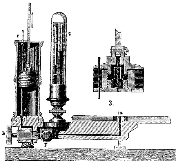
Черт. 2. Двухцилиндровая пневматическая машина в разрезъ.
