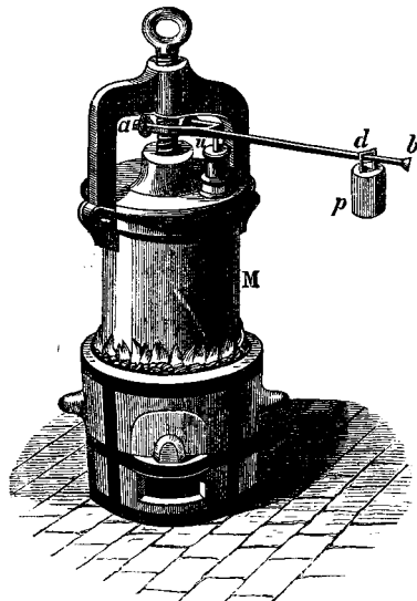
Папиновъ котель.
