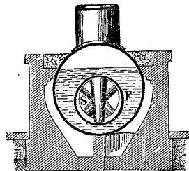
Котель Галловея.
