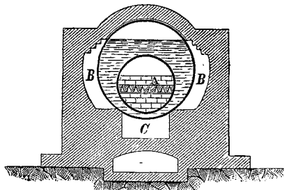
Корнваллійскій котель.
