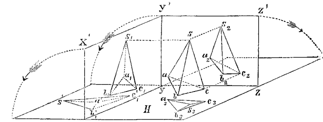
Начертательная геометрія.
