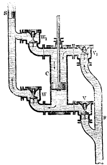
Насосъ Рнс. 2.
