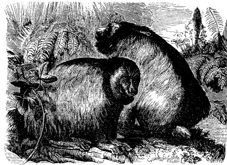
Brachyurus calvus .
