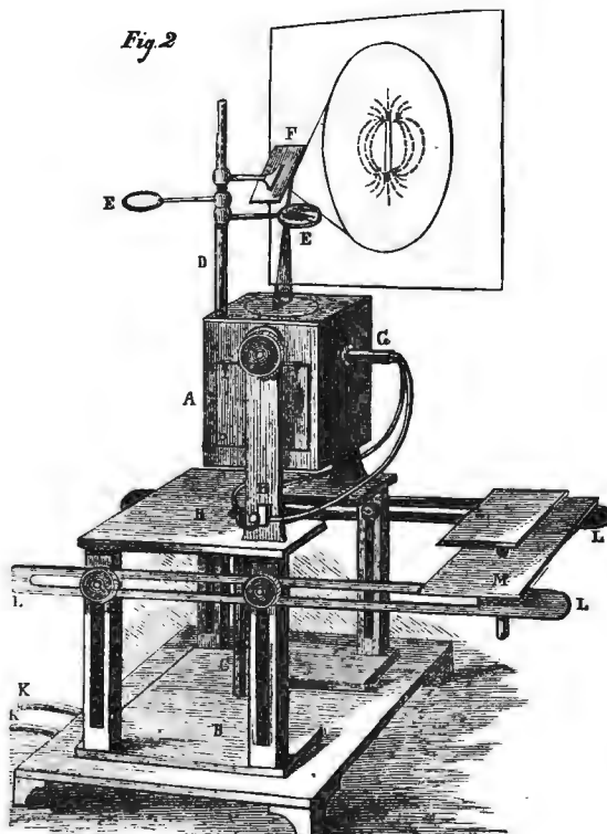
Намера-обскура, употребляемая при публичныхъ чтеніяхъ лекцій.
