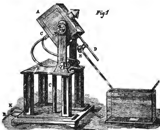
Намера-обскура, употребляемая при публичныхъ чтеніяхъ лекцій.
