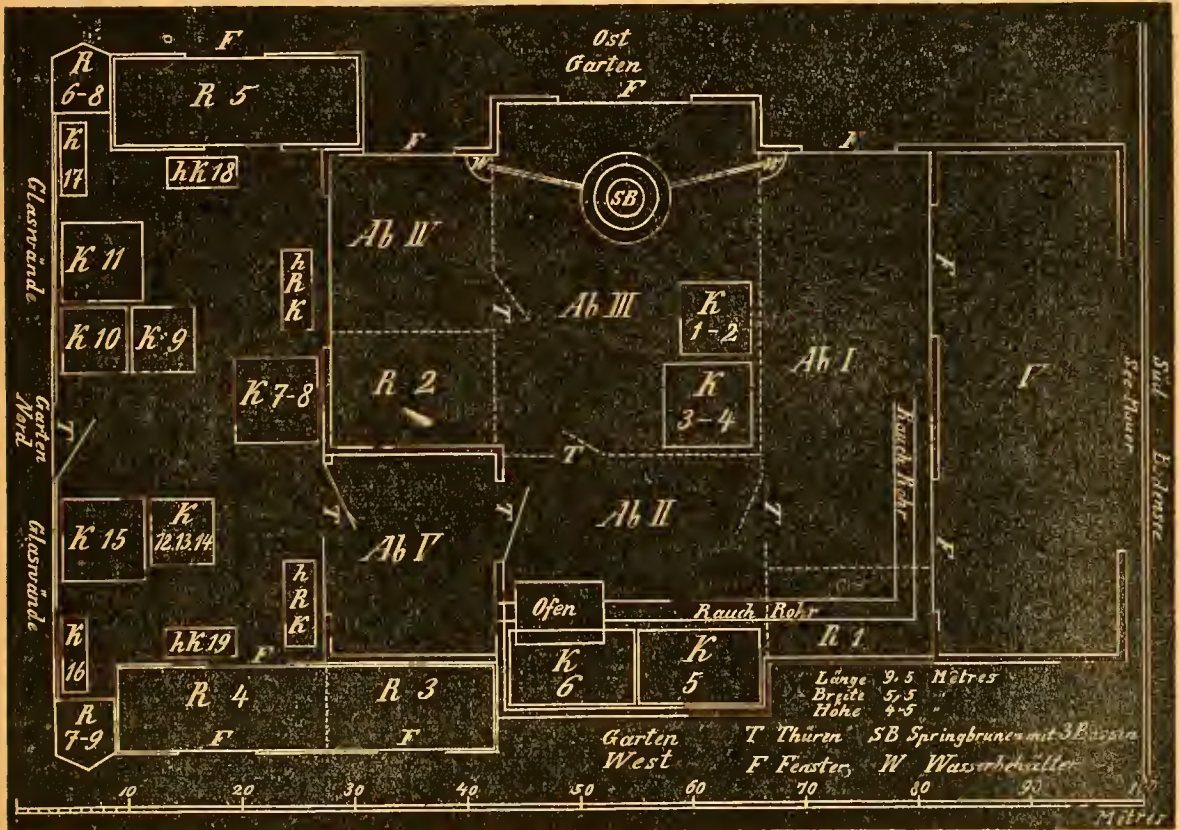
Vogelhaus des Herrn E. Linden in Radolfzell am Bodensee.
