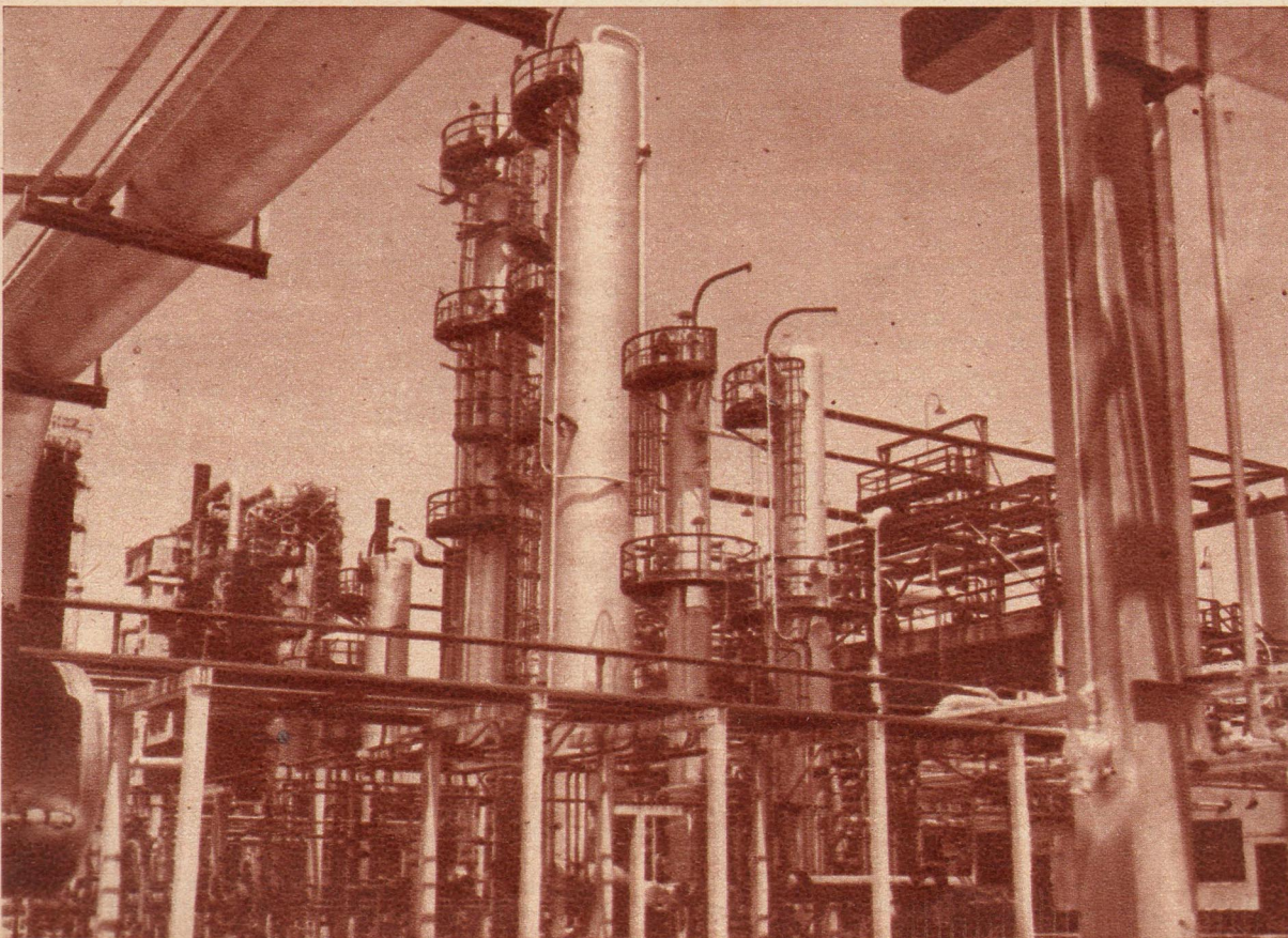
Una de las torres de elaboración de la destilería más grande de Sud América, próxima a inaugurarse.
