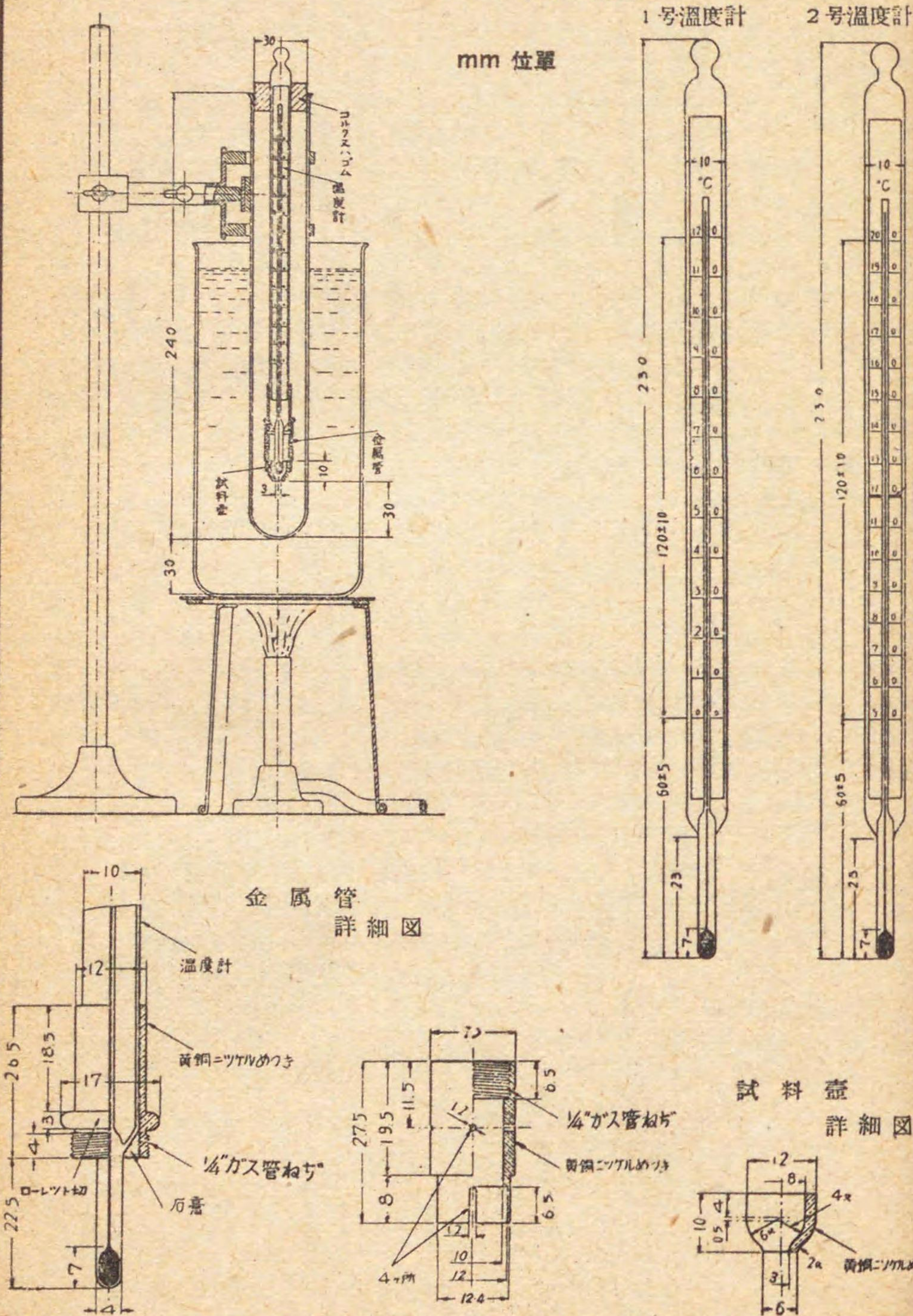
第 6 ウツペローテ式融点試験装置
