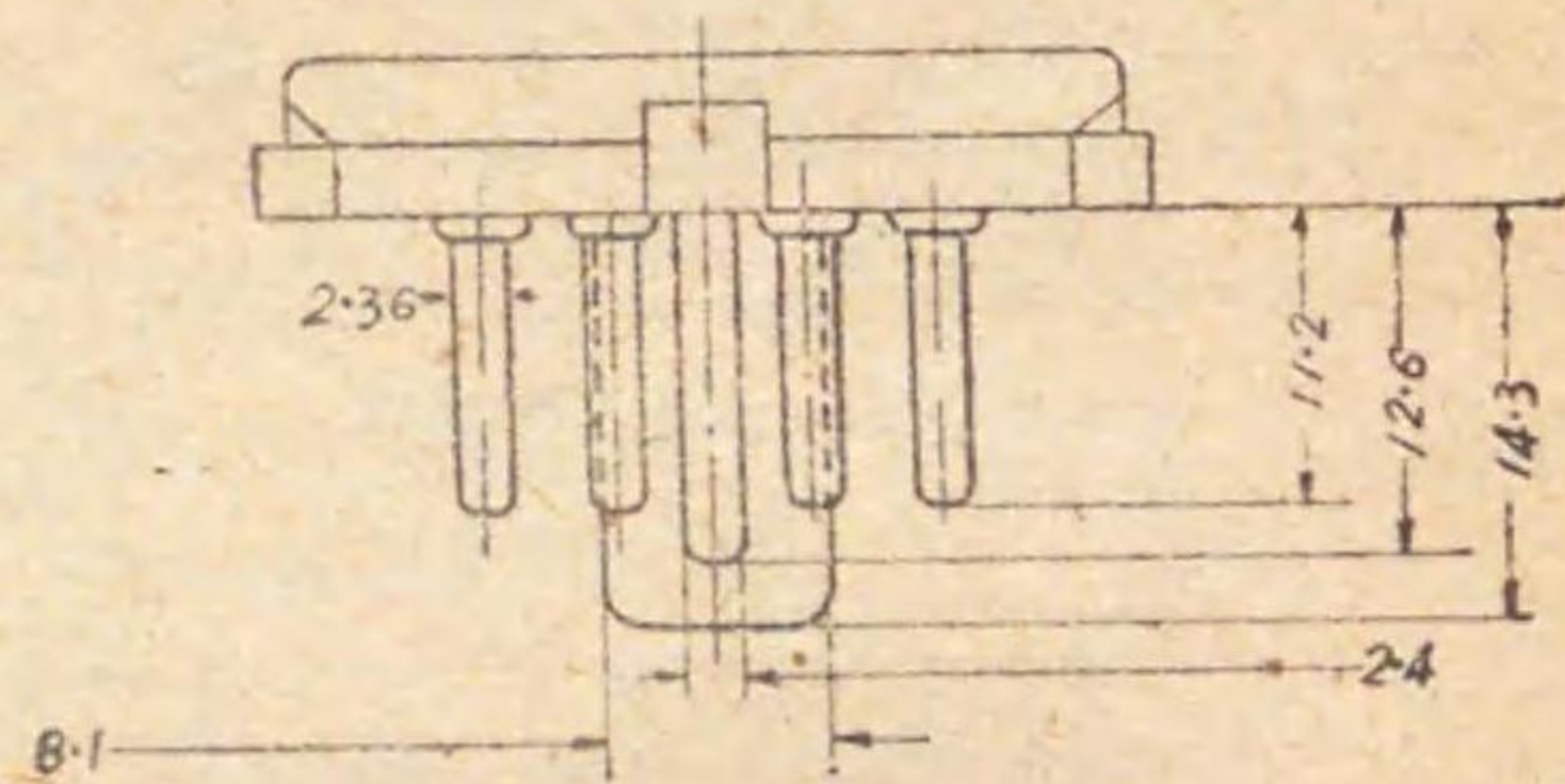
第 2 図 8 本脚用口金
