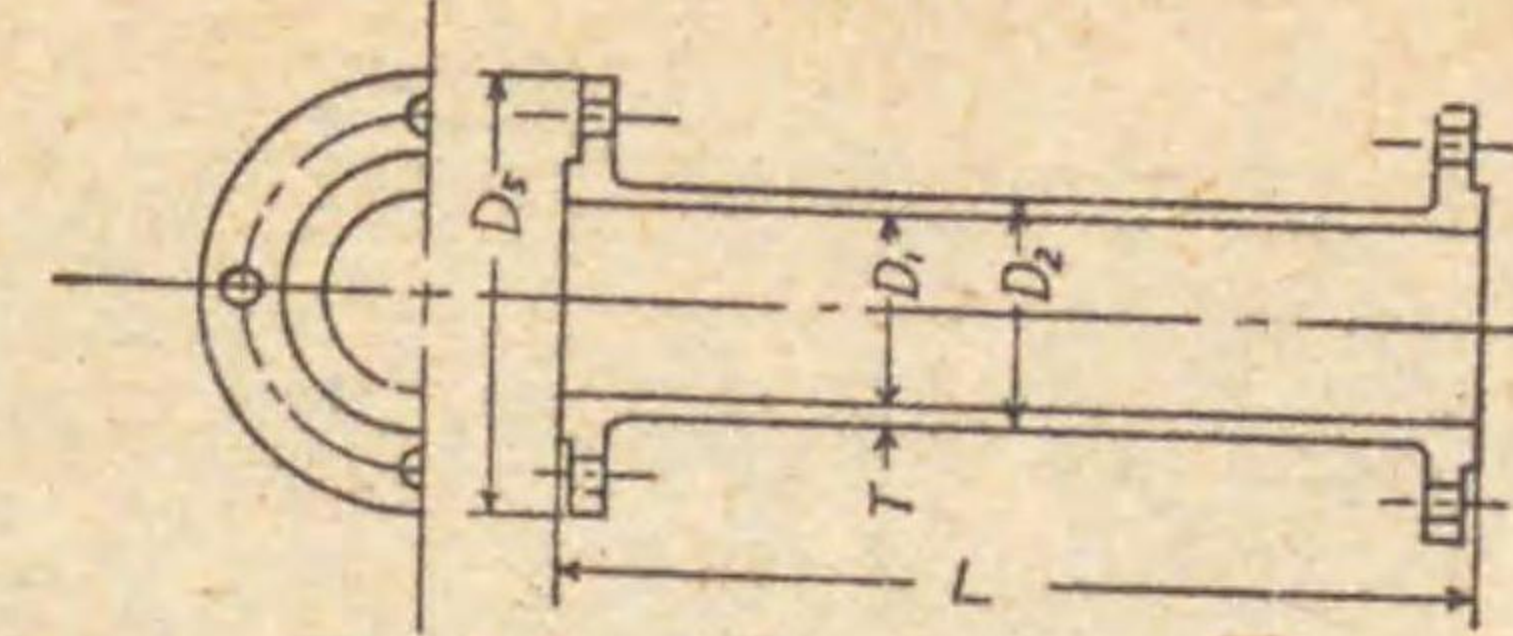
消火栓用管乙
