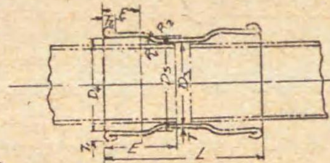
第十二号 接ぎ輪
