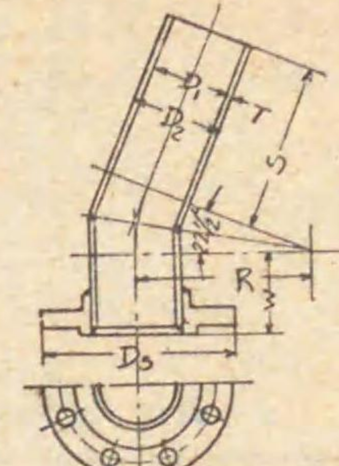
片鑄曲管 (22 1/2°) 單位 mm
