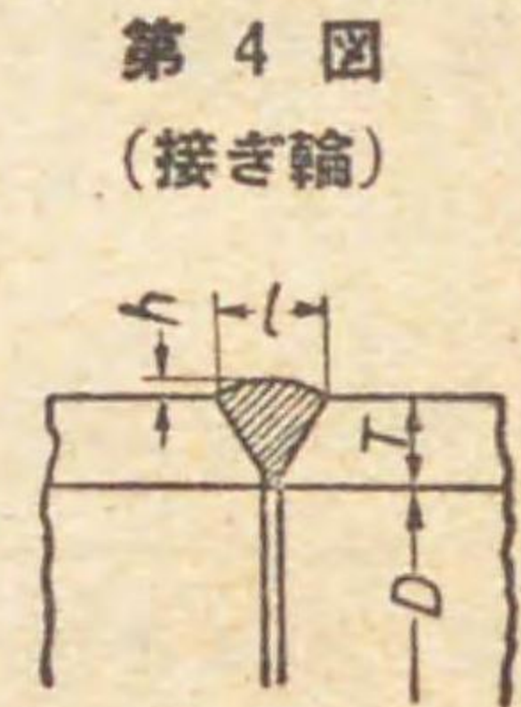
第 4 図 (接ぎ輪) l=1.2T 以上 h=0.2T 以上
