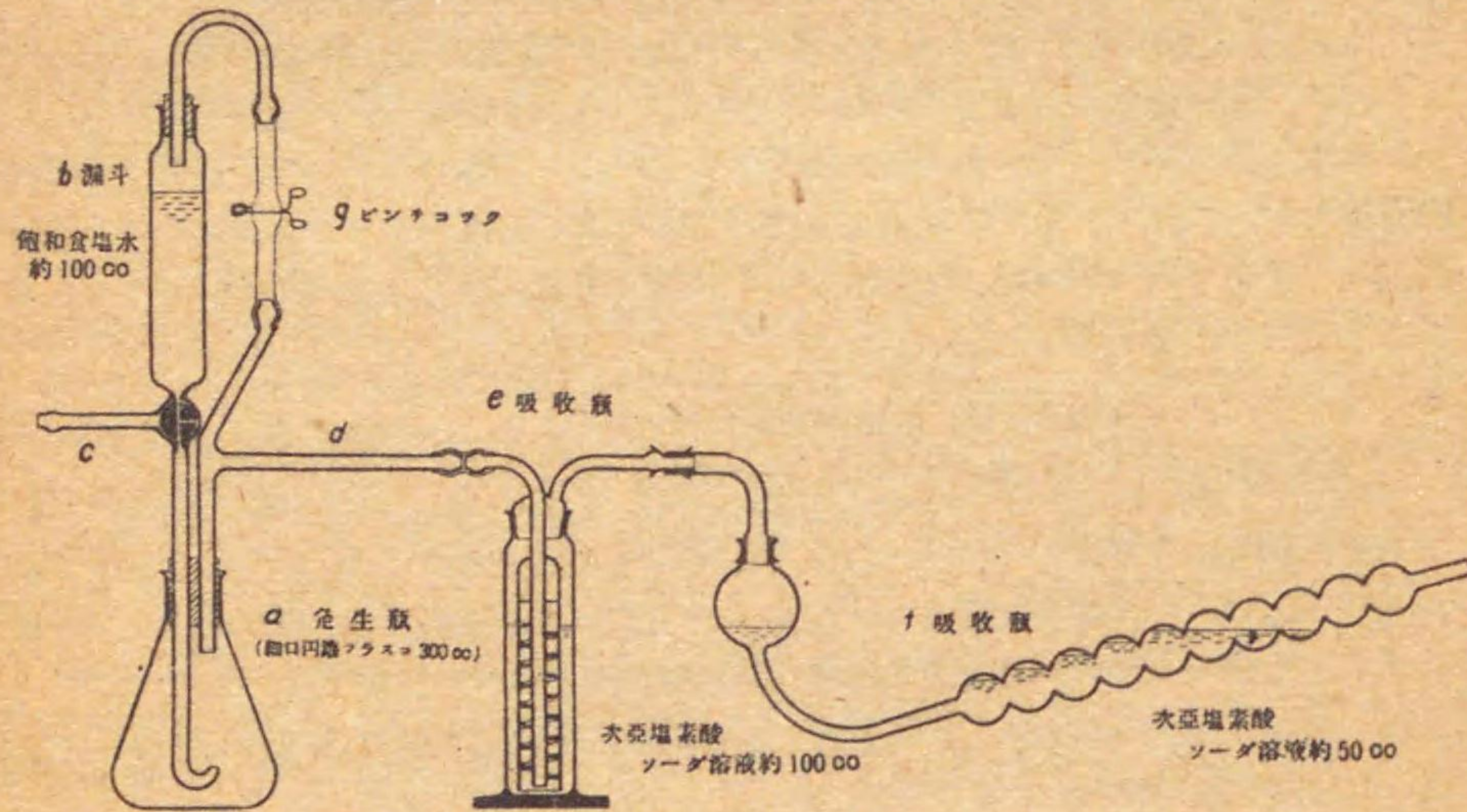
附図 燐化水素定量装置
