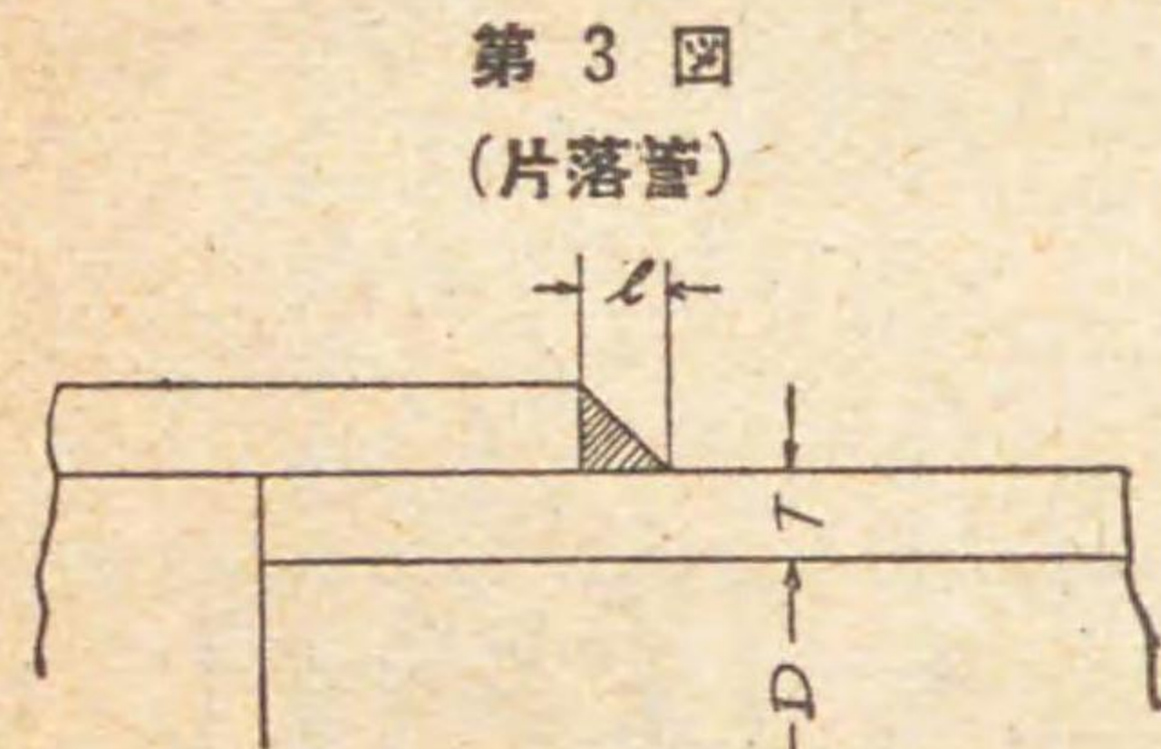
第 3 図 (片落管) l=T
