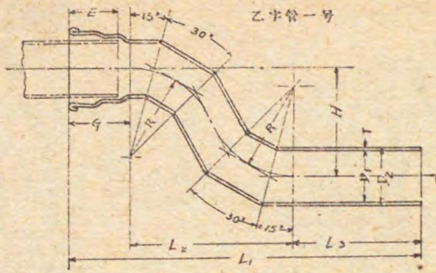
乙字管一号 單位 mm
