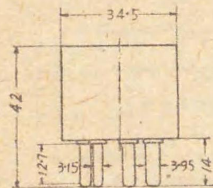
第 1 図 大型 7 本脚用口金
