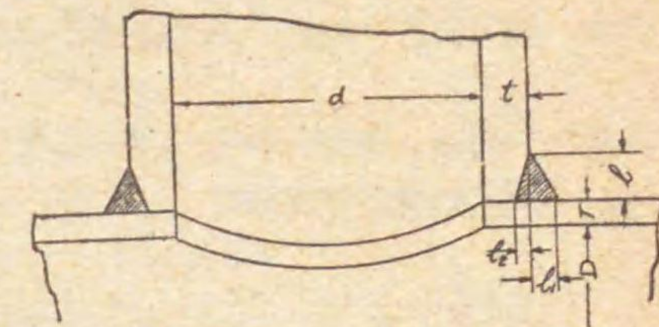
l=t 以上 h_1=T 以上 h_2=0.3t 以上
