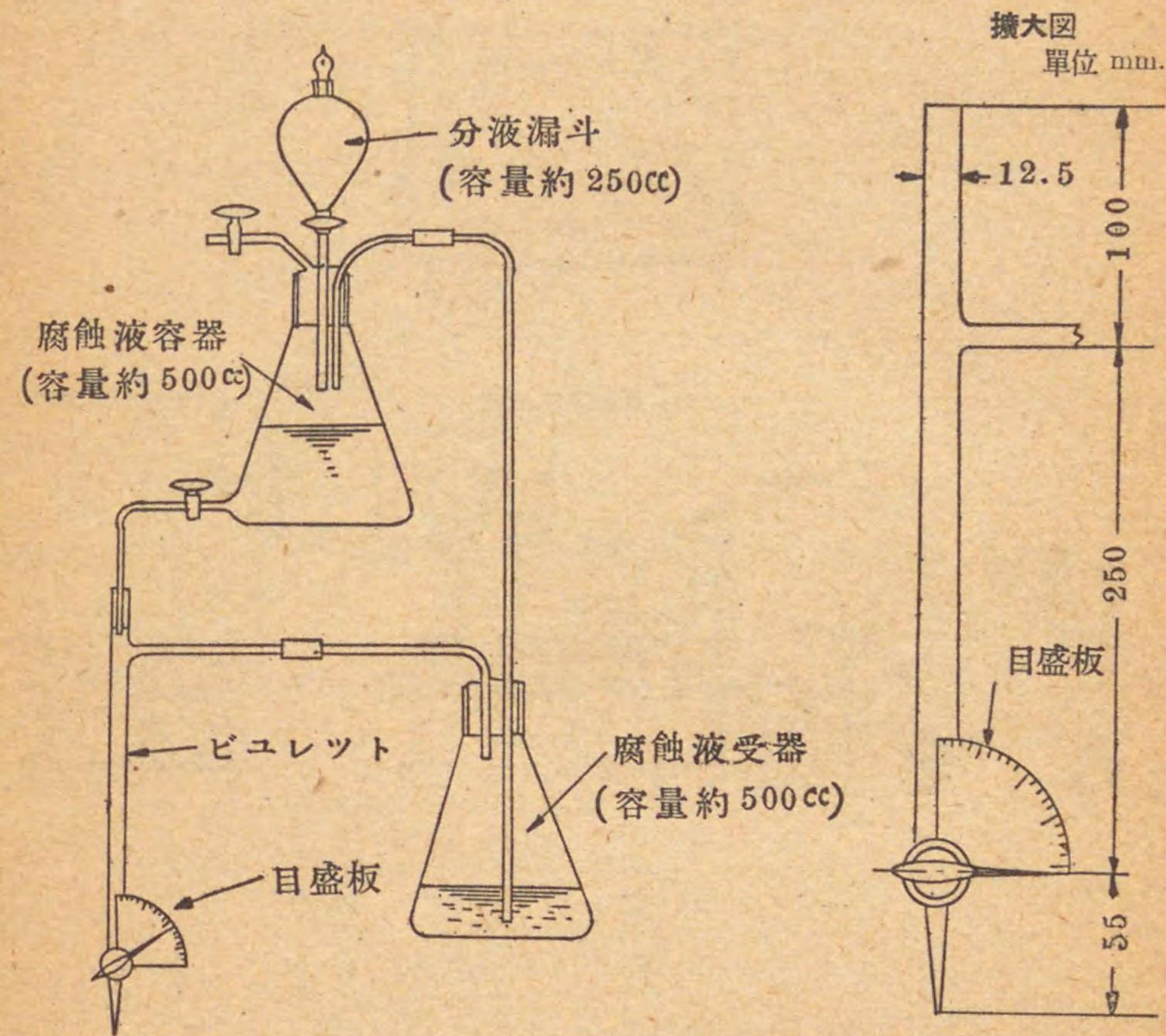
附圖第 1 腐蝕試験装置
