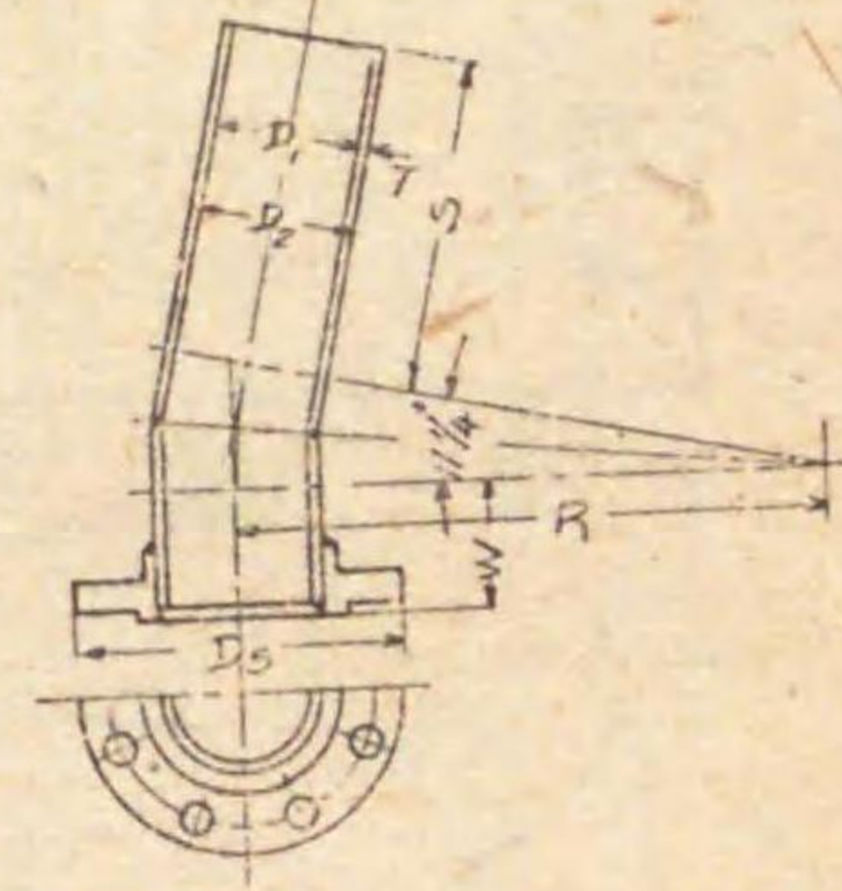
片鑄曲管 (11 1/4°) 單位 mm
