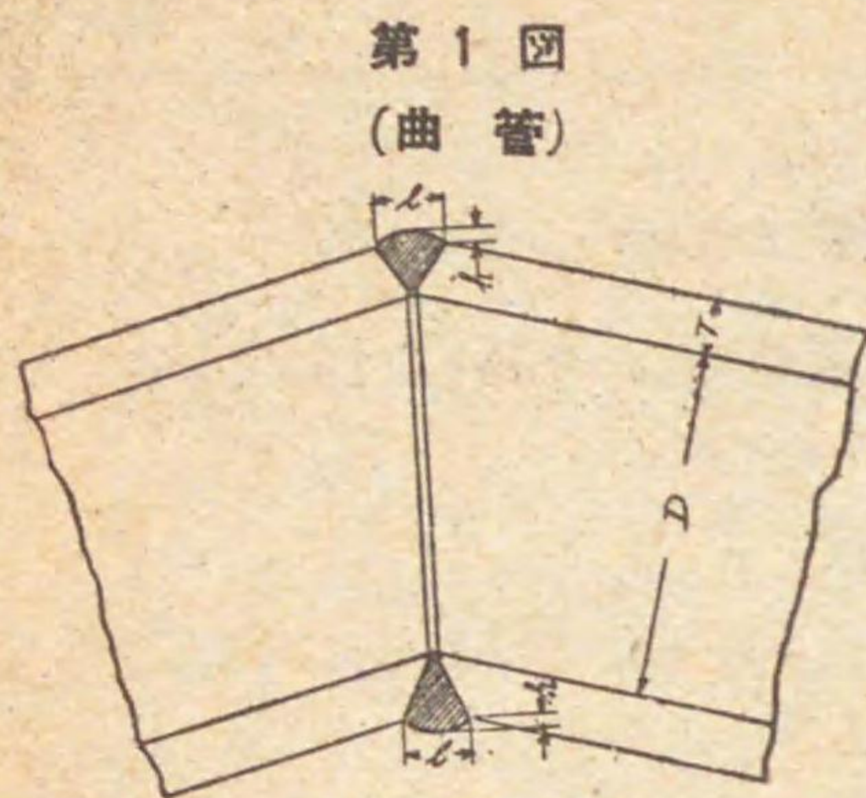
第 1 図 (曲管) h=0.2T 以上 l=1.2T 以上
