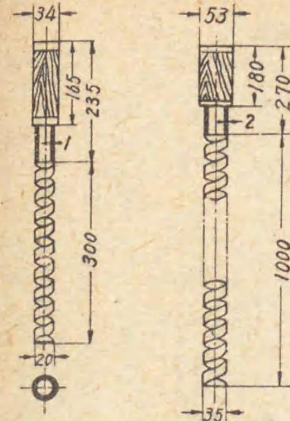
第 1 小型試料採取器 第 2 大型試料採取器
