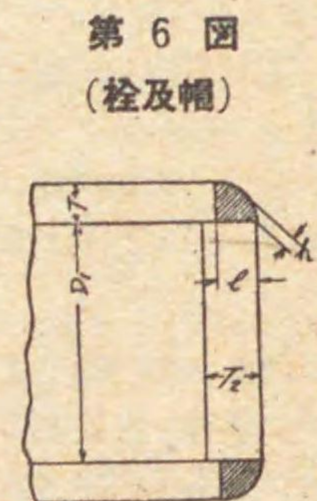
第 6 図 (栓及帽) h=T h=0.2T
