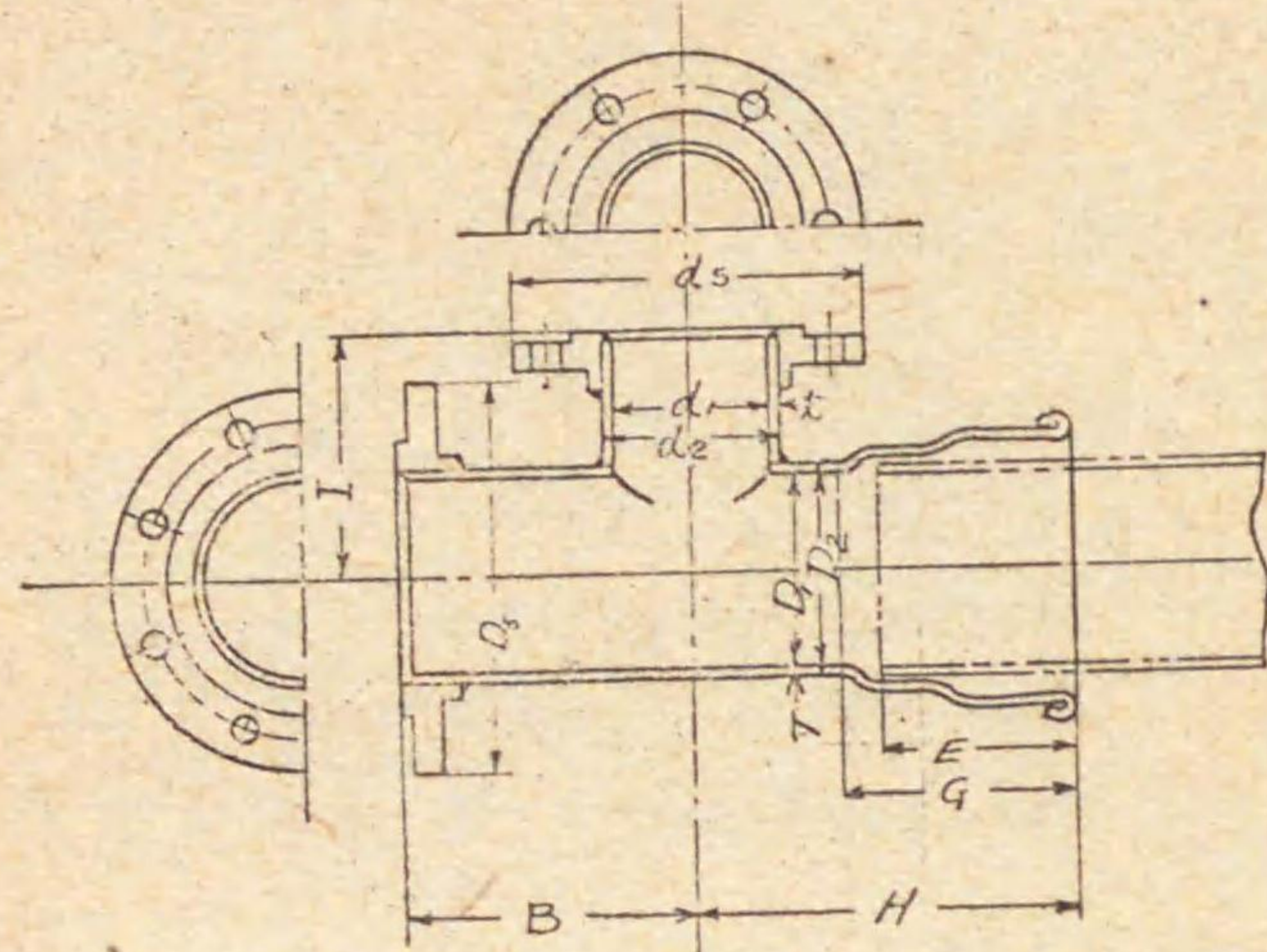
一受二銜丁字管
