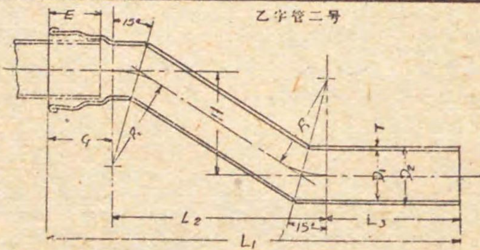
乙字管二号 單位 mm
