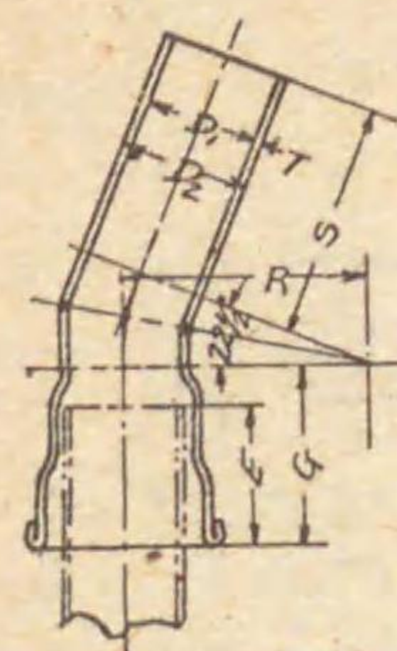
曲管 (22 1/2°) 單位 mm
