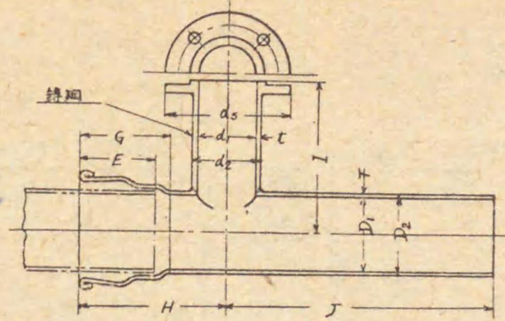
消火栓用管甲二号
