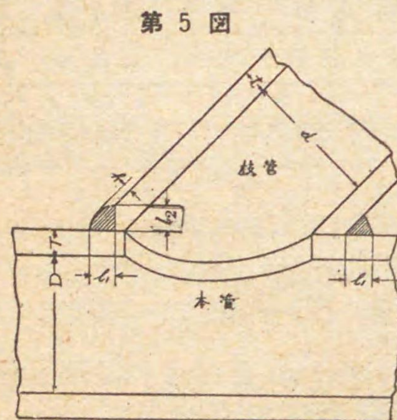
第 5 図 h_1=T 以上 h_2=T 以上 h=0.2T 以上
