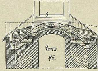
Фасады свода по стили станы Ж.
