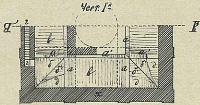
Планъ западной части свода.
