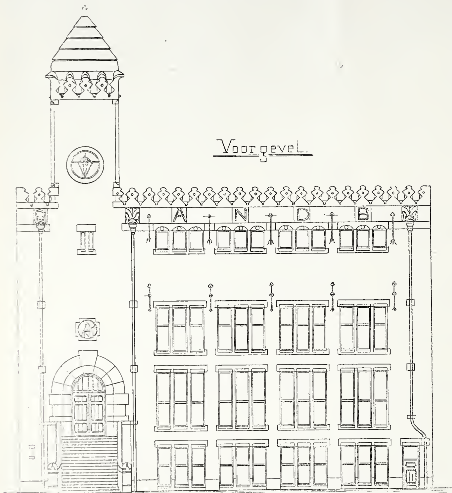
Schaal 1 à 200.
