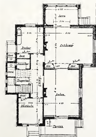
Beganegrond. Schaal 1 à 300.
