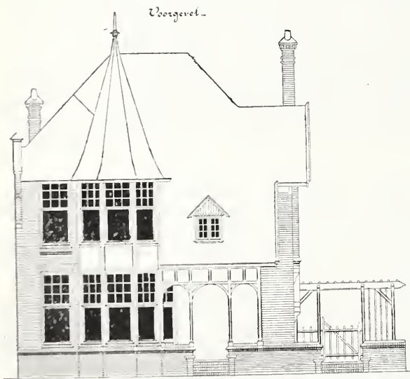
Schaal 1 à 200.
