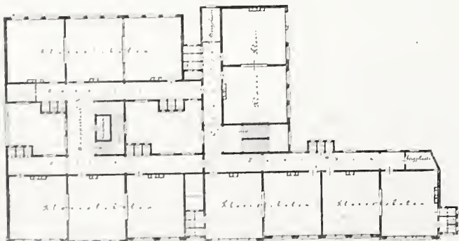
Eerste Verdieping. Schaal 1 à 600.
