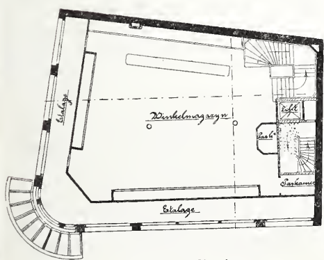
Eerste verdieping.
