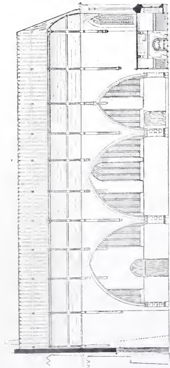
Doorsnede over de lengte, Schaal 1 à 100.
