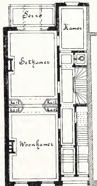
Hoog-parterre. Schaal 1 à 200.
