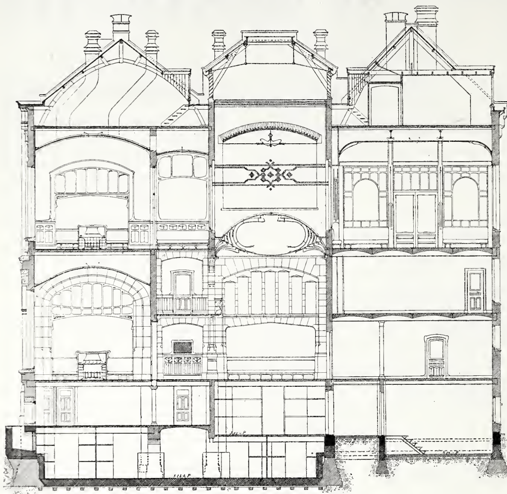
Doorsnede over AB. Schaal 1 à 200.
