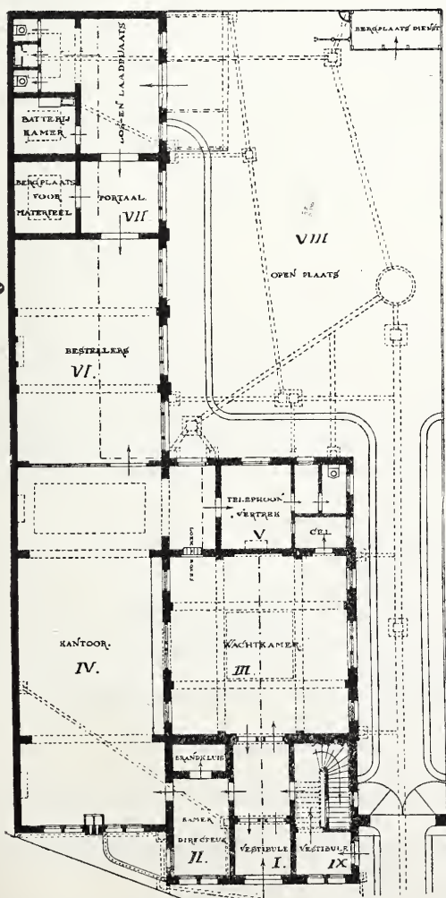
BEGANEGROUND. Schaal 1 à 300.
