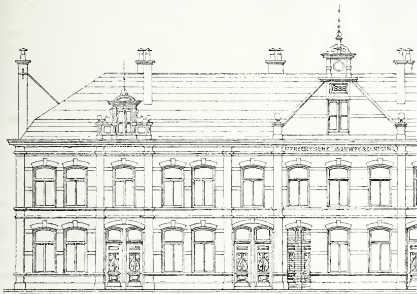
Woonhuizen met bovenwoning (9 in getal.)
