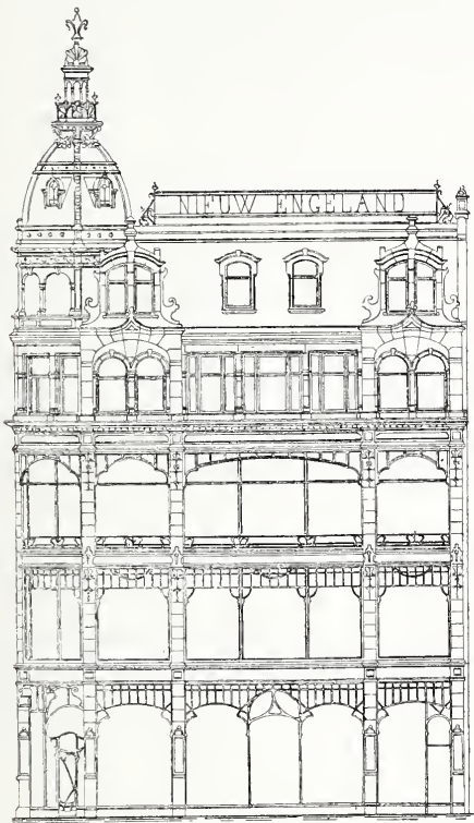
Gevel aan den Singel, hoek Koningsplein.
