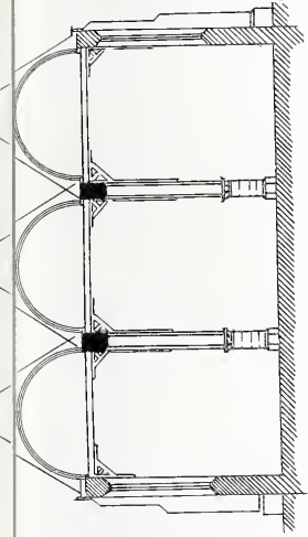
Doorsnede over de breedte. Schaal 1 à 400.
