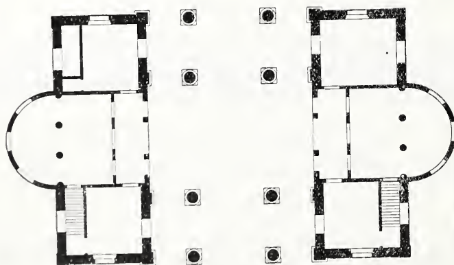
Plattegrond.
