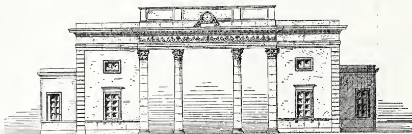
Gevel stadszijde.
