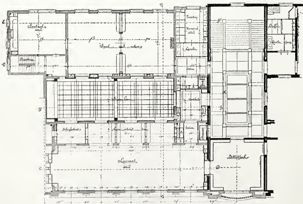
Eerste Verdieping. Schaal 1. à 300.
