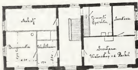
Verdieping. Schaal 1 à 300.
