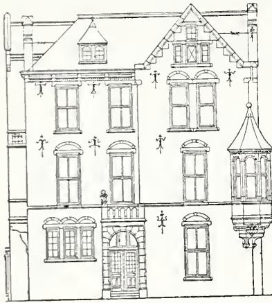
Gevel a/d. Laan van Meerderevoort. Schaal 1 à 300.
