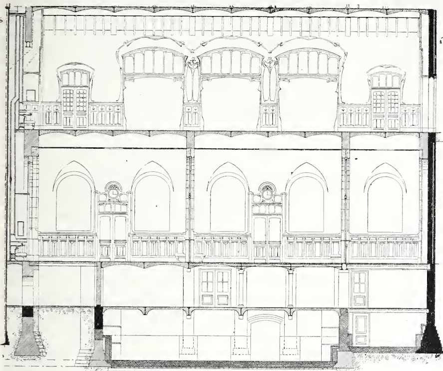
Doorsnede over C D. Schaal 1 à 200.
