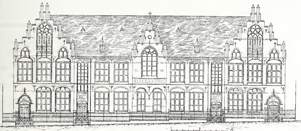
Gevel Sonsbeeksingel.
