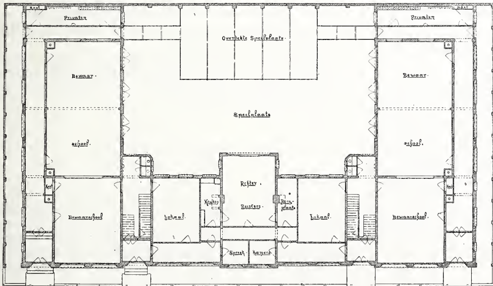
Beganegrond. Schaal 1 à 400.
