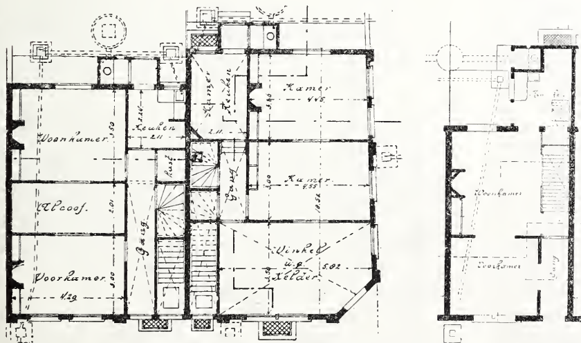
Woonhuis met bovenwoning. Winkelhuis. (7 in getal.)
