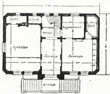
Hoofdverdieping. Schaal 1 à 300.
