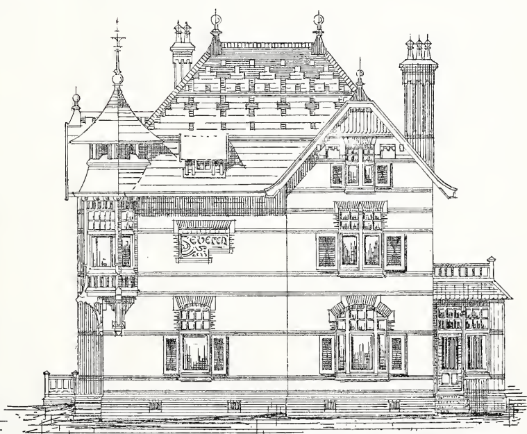
Zijgevel.
