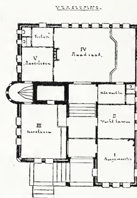
Schaal 1 à 400.
