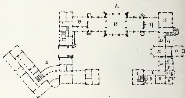
Eerste verdieping. Schaal 1 à 200.
