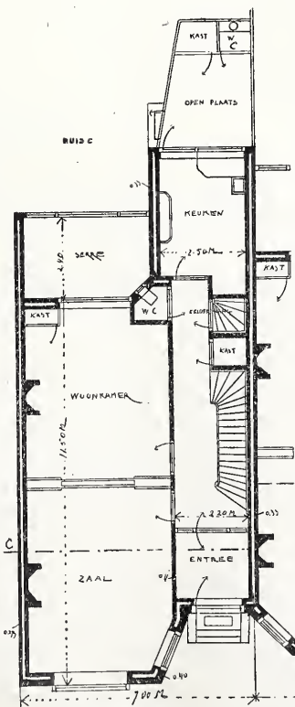
Plattegrond. Schaal 1 à 200.
