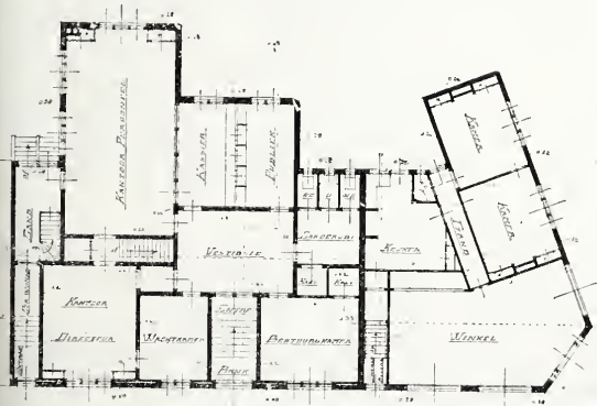
Plattegrond gelijkstraats. Schaal 1 à 400.
