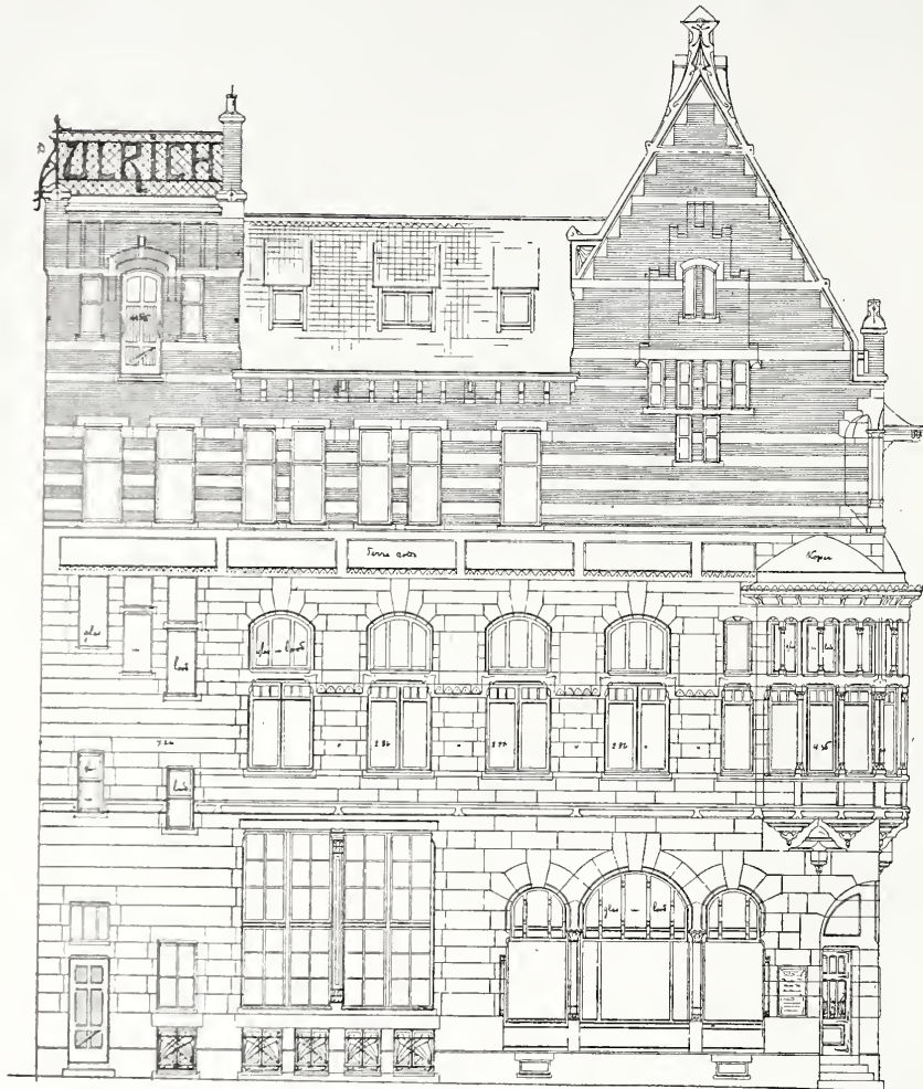
Gevel Leuvebrugsteeg.
