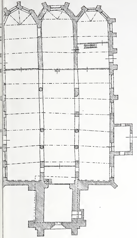
Plattegrond. Schaal 1 à 400.
