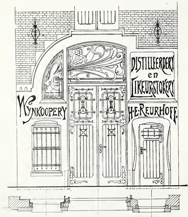
Schaal 1 à 60.
