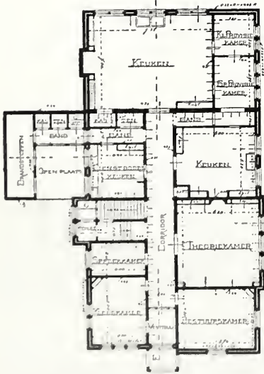
Plan v. d. Beganegrond. Schaal 1 à 400.
