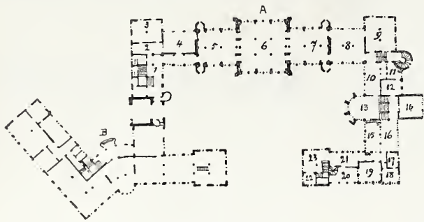
Beganegrond. Schaal 1 à 200.
