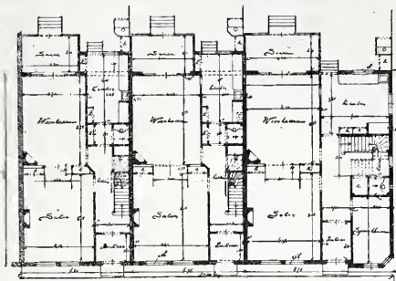
Plattegrond gelijkstraat. Schaal 1 à 400.
