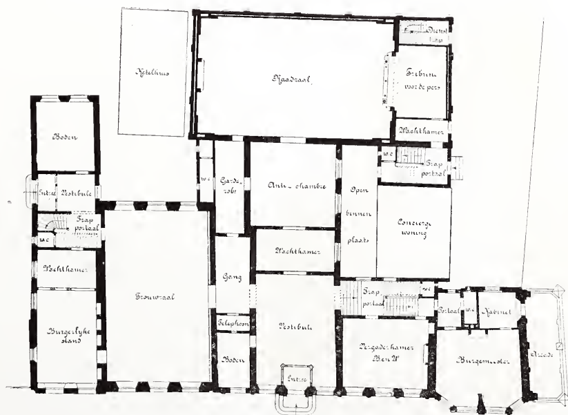
Plattegrond gelijkstraats. Schaal 1 à 400.
