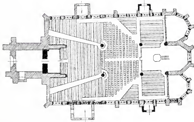
Plattegrond. Schaal 1 à 600.
