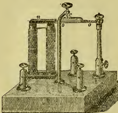
FIG. 12. WAGNER'S HAMMER.
