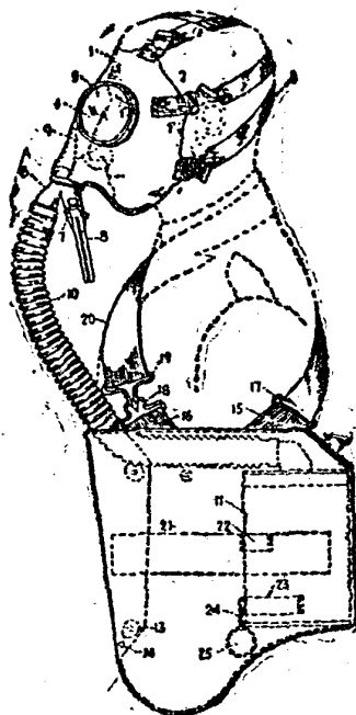
第一百圖 美國式軍用防毒面具
