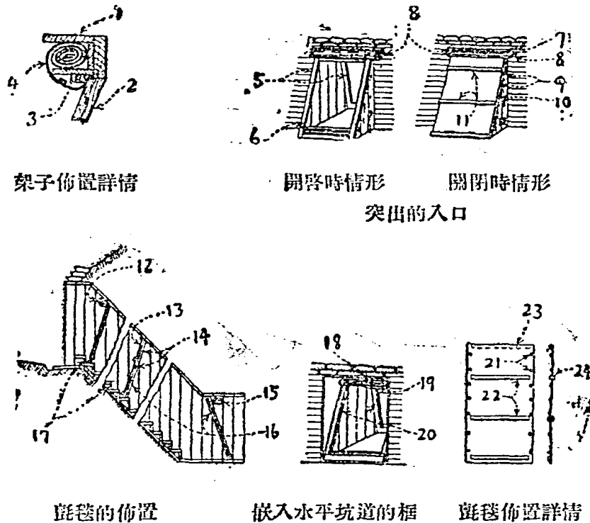
第一零一圖 地下防毒掩蔽部的佈置
