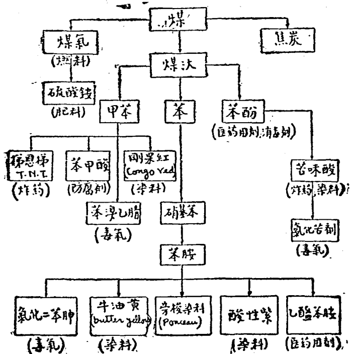
第一零四圖 由煤得出的產品 (平時及戰時)
