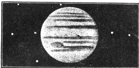
蓋利略在望遠鏡中所見的諸小月
