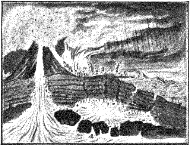
水從海底透過地殼，落入地中，地中的熱把牠化做水蒸氣。到後來氣體膨脹，將岩石炸裂。地裏面的熔石和熱泥，就出這裂口噴發出來。這種岩石的破裂，足以演成地震。圖中是畢壘火山口牠的爆裂大概就是這種原因。
