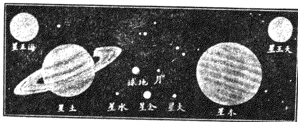
這是繞日諸行星的體積，可以看出他們的大小。比較木星的體積，地球要大一千二百倍。
