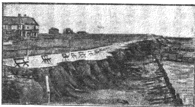
海濱衝去英國的海岸
