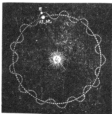
月和地球一樣的繞着太陽，不過牠不像地球的直繞，而同時又繞着地球的，看圖中所示便明。
