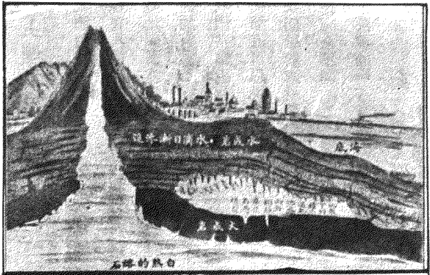
這圖表明火山爆發而為地震的原因看了這圖我們好像親見那大自然的機器正在準備演成那一齣慘劇一樣。圖中的火山雖還休息着，但去繼續噴火之期，已是不遠了。
