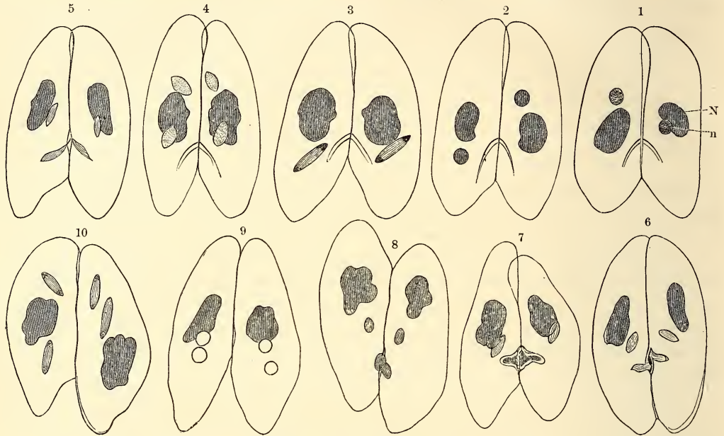
Population von Paramecium Aurelia . Schematisch.
