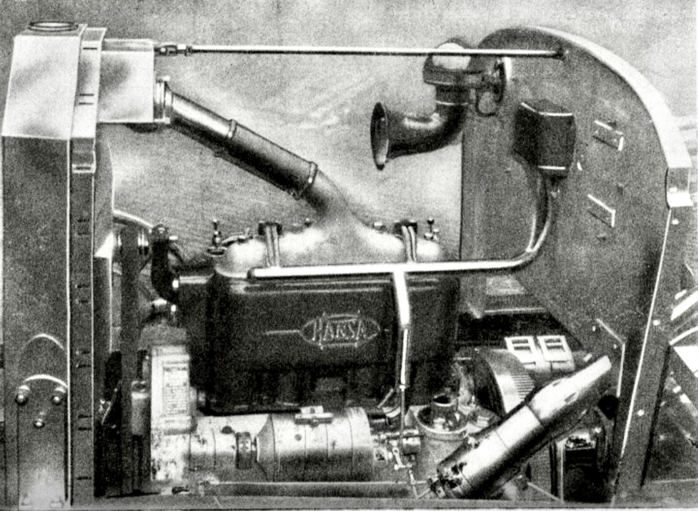
8 36 PS Hansa-Motor mit Lichtzündmaschine.
