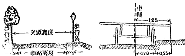
第二十二圖 步行道之寬度
