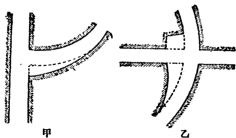
第十九圖 道路出口之加寬
