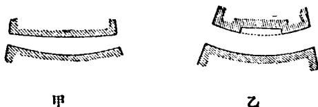
第二十圖 曲路之加寬
