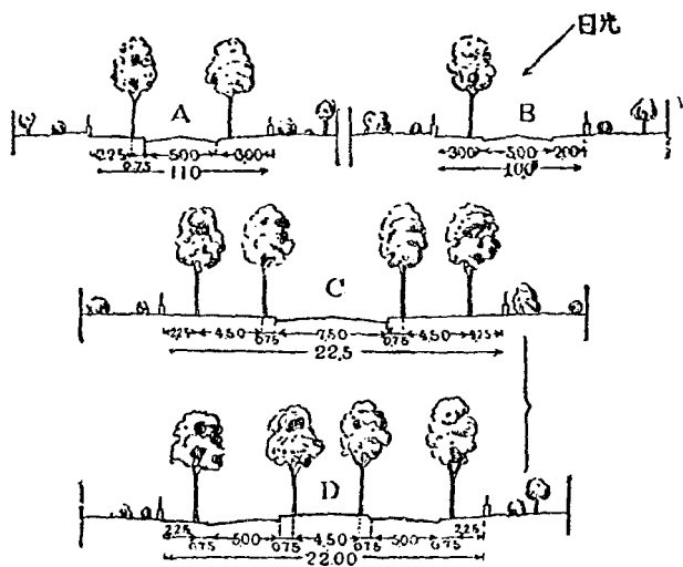
第二十五圖 居住區街道之寬度
