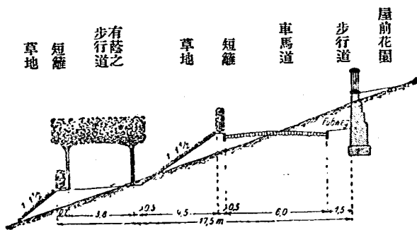
第三十一圖 德國邁仙市分離式山路
