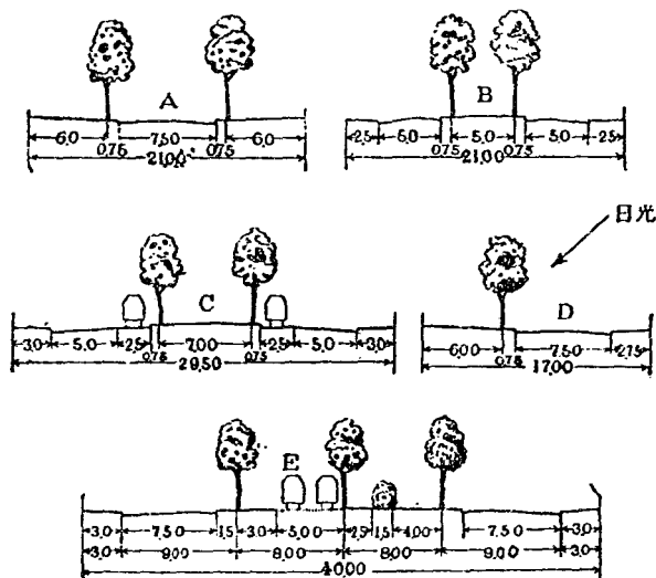
第二十四圖 街道之畫分路帶
