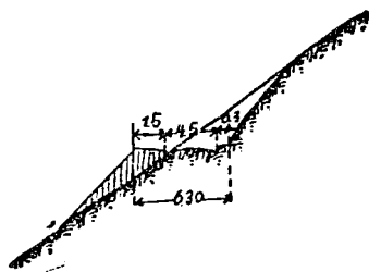
第二十九圖 山坡之路寬
