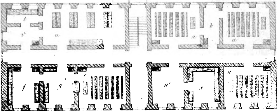
Кухенный этажъ.
