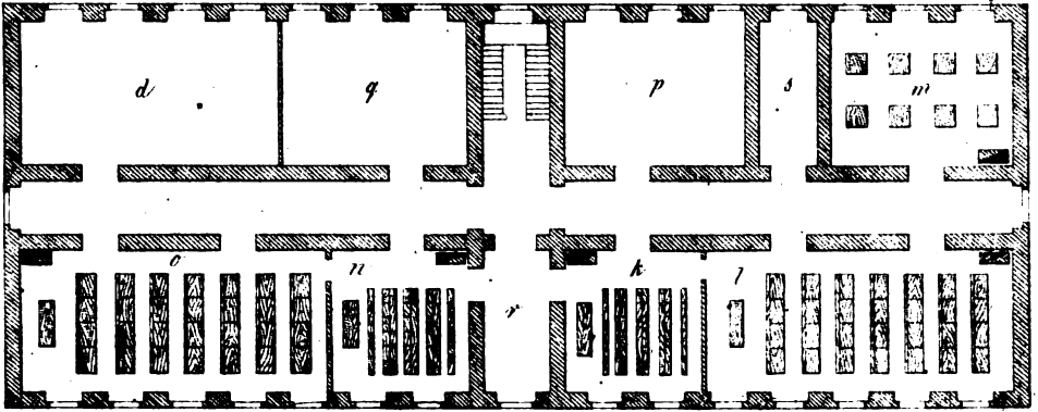
Второй этажъ.
