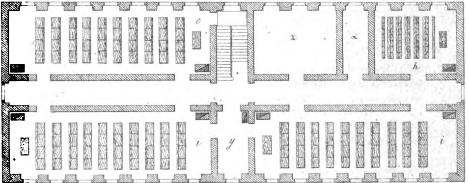
Кухенный этажъ.
