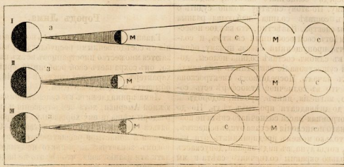
1) Мгновенное затмѣніе. 2) Затмѣніе полное продолжительное. 3) Затмѣніе кольцеобразное.
