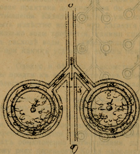
Рис. 2. Пара приствольныхъ круговъ съ частью разводящей воду борозды 0 и соединительными бороздками: а — кольцевая канавка, которая дѣлается вершковъ 8—7 ширины и 4 5 верш. глубины, d — дерево.
