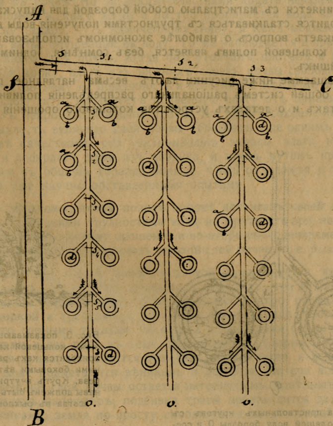
Рис. 1. Общій планъ оросительной системы. АВ и АС главныя, проводящія воду борозды. Переваливая борозду АС последовательно въ S, въ S1, S2, S3, можно направить воду въ борозды, идущія по междурядьямъ - O, O1, O2. Изъ каждой такой борозды вода проводится последовательно въ ab (или кольцевыя канавки при взрослыхъ деревьяхъ). Черточки указываютъ мѣста, въ которыхъ переваливается борозда, чтобы дать водѣ желаемое направленіе.
