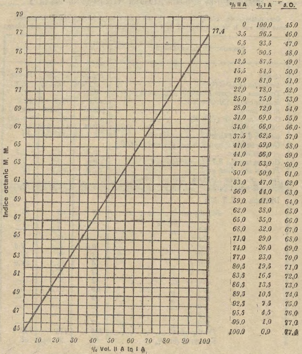
CURBA VALORILOR INDICELUI OCTANIC AL AMESTECURILOR DIN BENZINELE DE REFERINȚĂ I A ȘI II A METODA MOTOR
