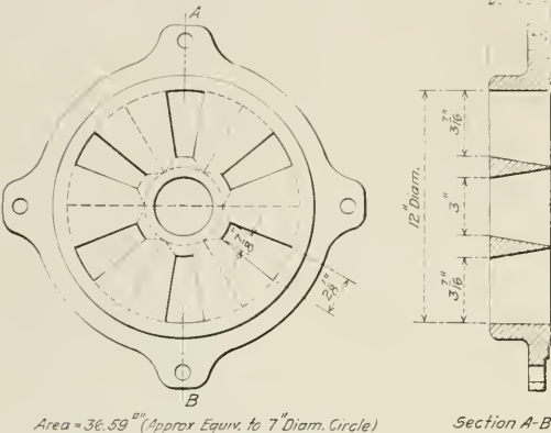
Fig. 6—Plain Annular Nozzle A-1
