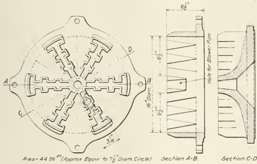
Fig. 14—Waffle Iron Nozzle A-5
