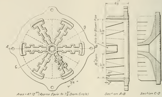
Fig. 21—Waffle Iron Nozzle A-10
