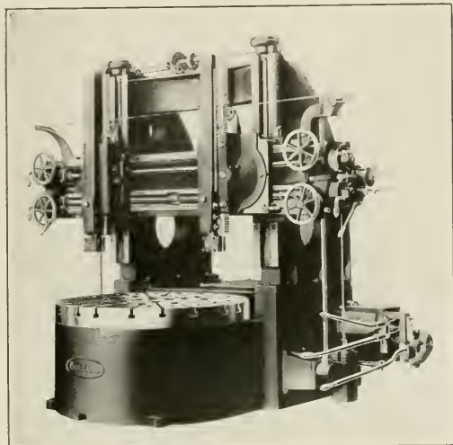
Fig. 1—Bullard 61-In. Maxi-Mill
