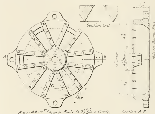
Fig. 12—Annular Nozzle A-4
