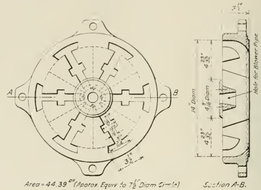
Fig. 8—Waffle Iron Nozzle A-2
