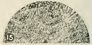
Fig. 15—Test Piece 15—1200 Dia.
