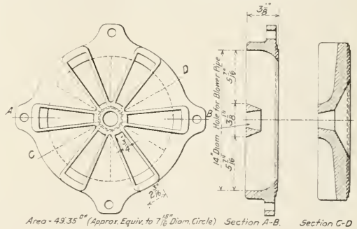
Fig. 23—Annular Nozzle A-4b
