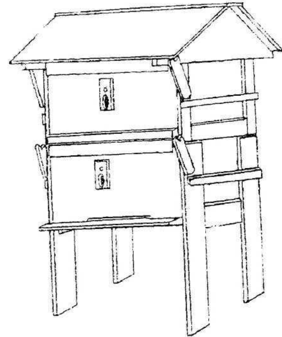
Рис. № 1. Алтайскій улей спереди и слева въ положеніи для времени главного сбора. Около 1/2 натуральной величины.
